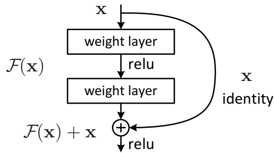
Figura 37 – Bloco Residual: x contorna as camadas intermediárias F(x) via uma função identidade somando-se a própria F(x) ao final do bloco.
