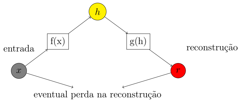
Figura 33 – Representação funcional de um autoencoder : Sendo o vetor x uma entrada, então o vetor h é estado resultante da aplicação de uma função codificadora f sobre x : h = f(x) , portanto r é a reconstrução de x a partir h através de uma função decodificadora g : r = g(h) . Tal processo pode ou não implicar em uma perda de informação.
