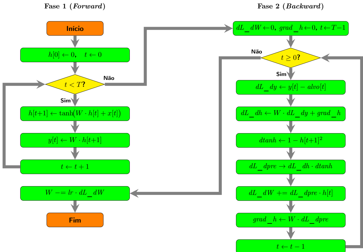
Figura 29 – Fluxograma do algoritmo BPTT simplificado. Fase 1 ( forward ): computa e armazena h[t] e y[t] para cada passo t . Fase 2 ( backward ): percorre os passos em ordem inversa, acumula o gradiente \partial\mathcal{L}/\partial W e propaga grad\_h para a etapa anterior.
