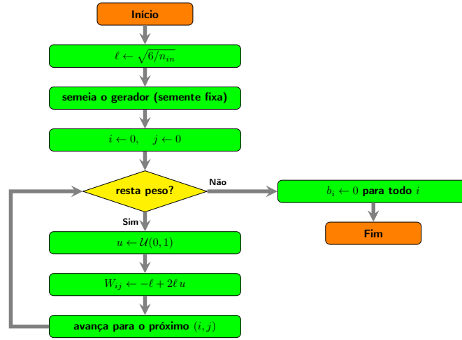
Figura 32 – Fluxograma da inicialização de He/Kaiming: calcula-se o limite \ell , semeia-se o gerador, percorrem-se todos os pesos sorteando cada um em [-\ell, +\ell] e, ao final, zeram-se os vieses.
