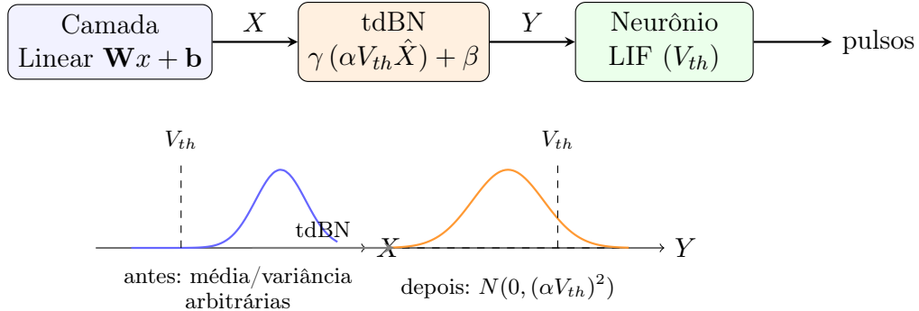
Figura 30 – Normalização em Lote Dependente do Limiar (tdBN): inserida entre a camada Linear e o neurônio LIF, ela agrupa as estatísticas sobre lote e tempo e reescala a corrente para a distribuição N(0, (\alpha V_{th})^2) , mantendo uma fração controlada de neurônios acima do limiar V_{th} a cada passo.
