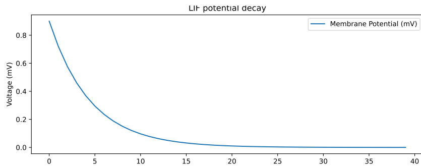
Figura 25 – Decaimento do potencial da membrana.
