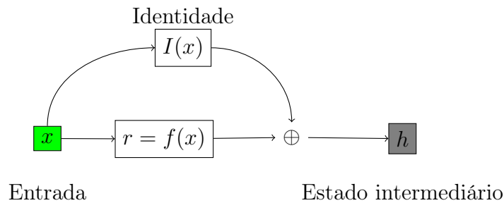
Figura 39 – Obtenção do resíduo: Se x é um vetor de entrada na rede e I(\cdot) é uma função identidade cujo valor é diretamente somado \oplus com o resultado produzido pelas várias camadas representadas por f(\cdot) , h é um vetor representando um estado intermediário de uma rede neural.
