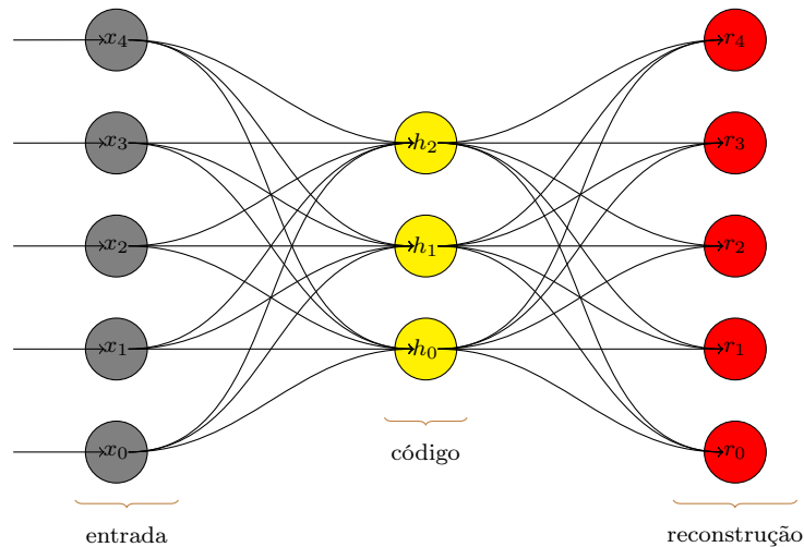
Figura 34 – Exemplo esquemático de um autoencoder sub-completo ou clássico: Os nós de entrada estão em cinza, a camada de código em amarelo contém as características codificadas e finalmente a camada de reconstrução em vermelho contém uma cópia aproximada da entrada.
