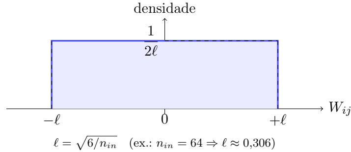
Figura 31 – Distribuição uniforme dos pesos na inicialização de He/Kaiming: cada peso é igualmente provável dentro de [-\ell, +\ell] , com \ell = \sqrt{6/n_{in}} , e densidade constante igual a 1/(2\ell) .
