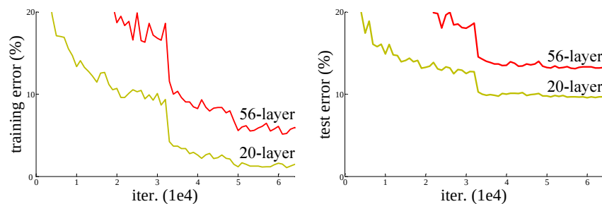
Figura 38 – Desempenho de duas redes neurais não residuais com 56 e 20 camadas. A esquerda a taxa de erro durante o treinamento, a direita a taxa de erro em relação ao conjunto de testes.
