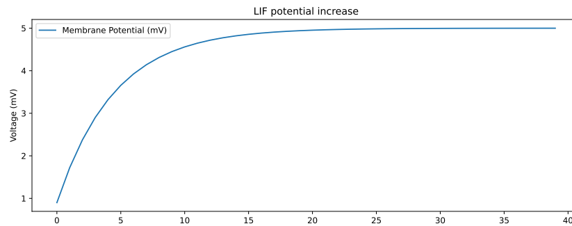
Figura 26 – Aumento do potencial da membrana.
