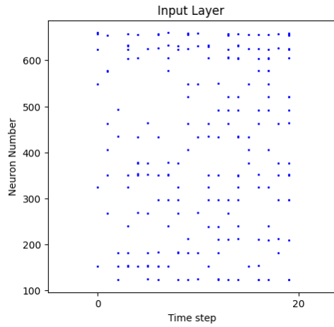
Figura 23 – Atividade dispersa de uma simulação RNP: O eixo horizontal representa o momento no qual os dados estão sendo processados e o vertical representa o número do neurônio (índice) na RNP. Note que, na maior parte do tempo, muito poucos neurônios são ativados.
