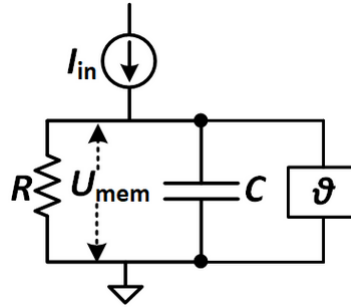
Figura 21 – O modelo RC
