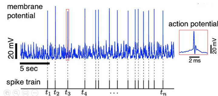
Figura 20 – Sinal ruidoso e os respectivos pulsos produzidos, note que é necessário um acúmulo de sinal suficiente antes que os pulsos comecem a ser exibidos
