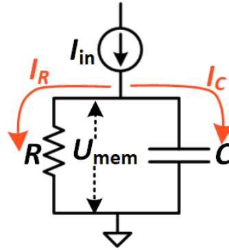
Figura 24 – Modelo RC para correntes: I_{in} = I_R + I_C
