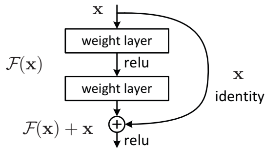
Figura 38 – Bloco Residual: x contorna as camada intermediárias F(x) via uma função identidade somando-se a própria F(x) ao final do bloco.
