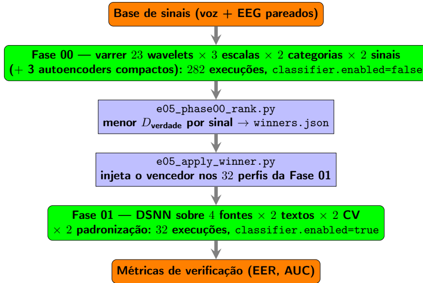
Figura 43 – Encadeamento das duas fases e dos scripts de transição
