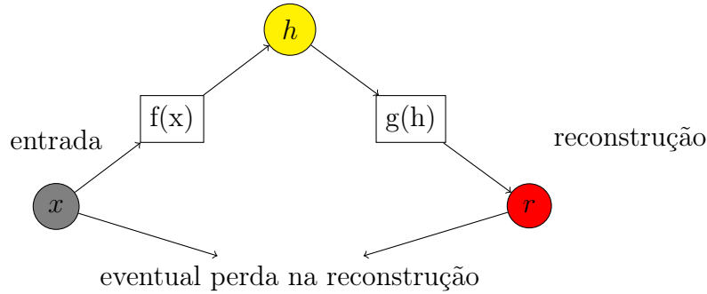
Figura 24 – Representação funcional de um autoencoder : Sendo o vetor x uma entrada, então o vetor h é estado resultante da aplicação de uma função codificadora f sobre x : h = f(x) , portanto r é a reconstrução de x a partir h através de uma função decodificadora g : r = g(h) . Tal processo pode ou não implicar em uma perda de informação.
