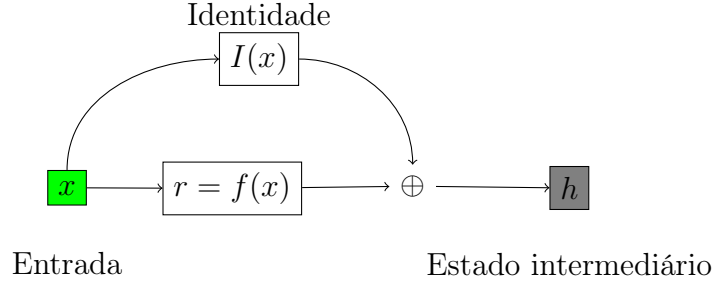
Figura 30 – Obtenção do resíduo: Se x é um vetor de entrada na rede e I(\cdot) é uma função identidade cujo valor é diretamente somado \oplus com o resultado produzido pelas várias camadas representadas por f(\cdot) , h é um vetor representando um estado intermediário de uma rede neural.
