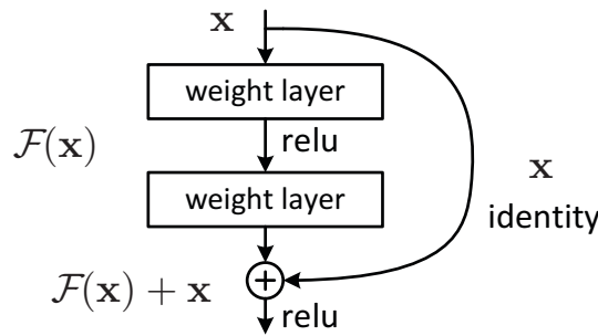
Figura 37 – Bloco Residual: x contorna as camadas intermediárias F(x) via uma função identidade somando-se a própria F(x) ao final do bloco.
