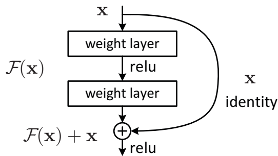
Figura 38 – Bloco Residual: x contorna as camadas intermediárias F(x) via uma função identidade somando-se a própria F(x) ao final do bloco.
