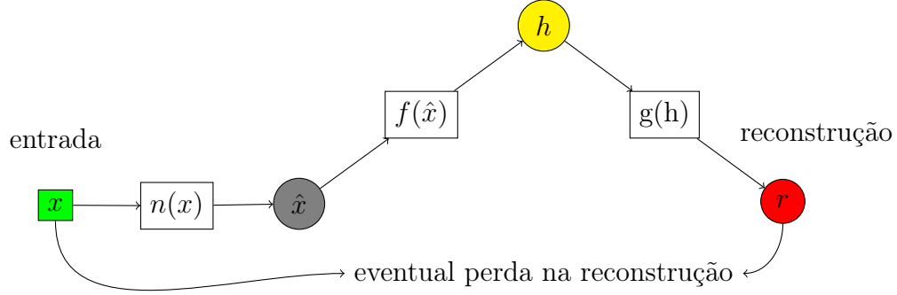
Figura 34 – Representação funcional de um denoising autoencoder : Sendo o vetor x uma entrada e n um função que adiciona um ruído aleatório então a informação com ruído \hat{x} é definida como \hat{x} = n(x) , portanto o vetor h é resultado da aplicação de uma função codificadora f sobre x : h = f(x) , finalmente r é a reconstrução de x a partir h através de uma função decodificadora g : r = g(h) . É importante notar que r é comparada com x e não com \hat{x} .
