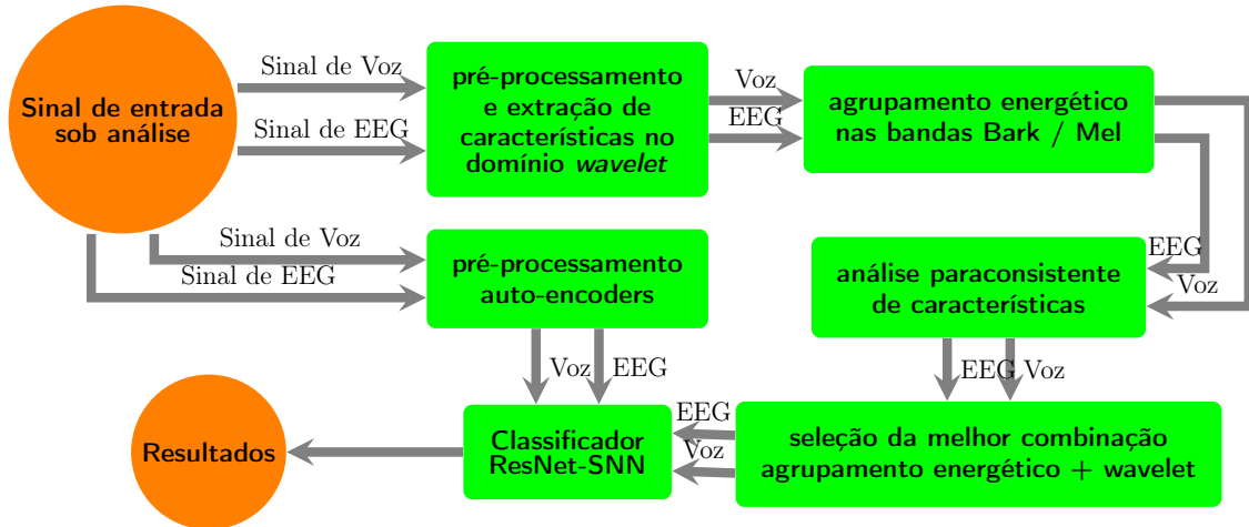
Figura 39 – Fluxograma da estratégia proposta
