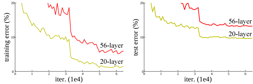
Figura 36 – Desempenho de duas redes neurais não residuais com 56 e 20 camadas. A esquerda a taxa de erro durante o treinamento, a direita a taxa de erro em relação ao conjunto de testes.
