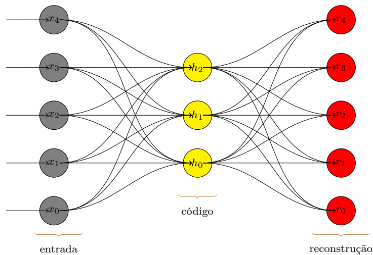
Figura 32 – Exemplo esquemático de um autoencoder sub-completo ou clássico: Os nós de entrada estão em cinza, a camada de código em amarelo contém as características codificadas e finalmente a camada de reconstrução em vermelho contém uma cópia aproximada da entrada.
