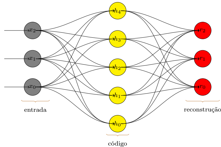
Figura 33 – Exemplo esquemático de um autoencoder supra-completo.
