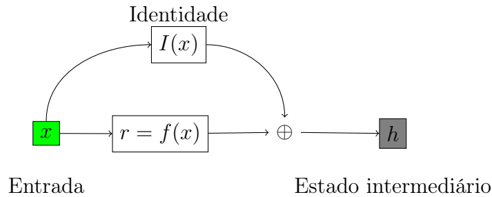
Figura 37 – Obtenção do resíduo: Se x é um vetor de entrada na rede e I(\cdot) é uma função identidade cujo valor é diretamente somado \oplus com o resultado produzido pelas várias camadas representadas por f(\cdot) , h é um vetor representando um estado intermediário de uma rede neural.
