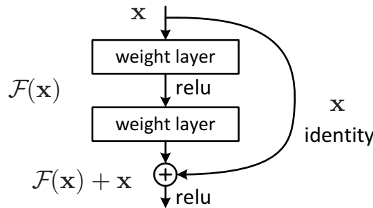
Figura 35 – Bloco Residual: x contorna as camada intermediárias F(x) via uma função identidade somando-se a própria F(x) ao final do bloco.
