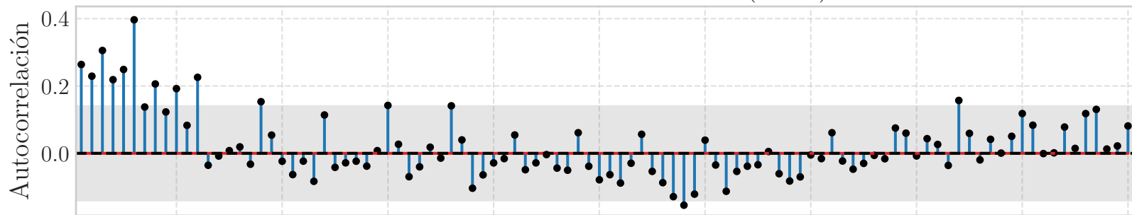
Función de Autocorrelación (ACF)
