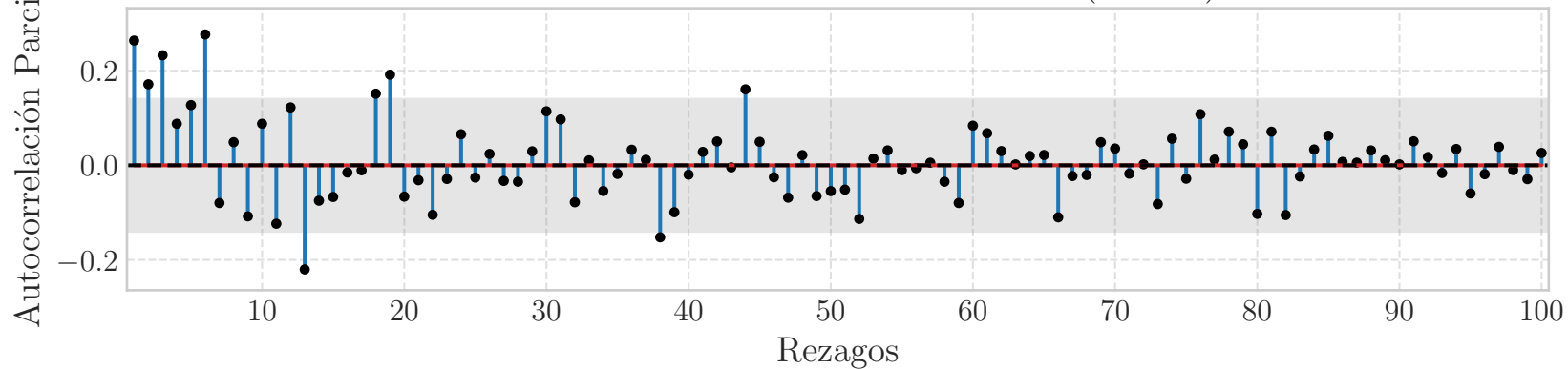
Función de Autocorrelación Parcial (PACF)
