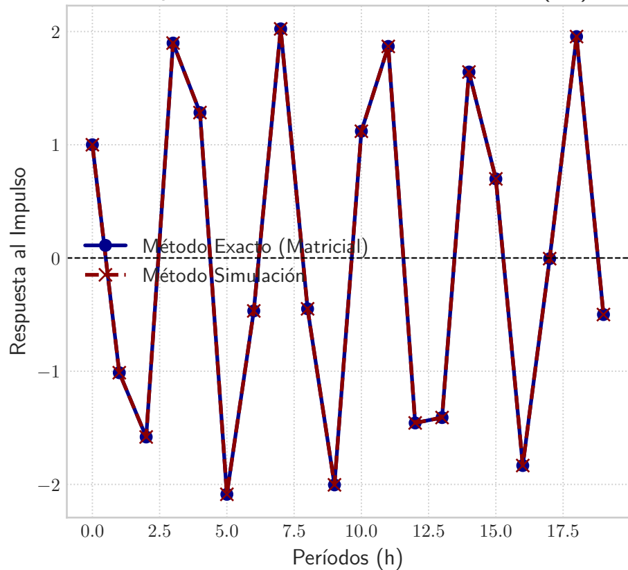
Comparación IRF de un Proceso AR(20)
