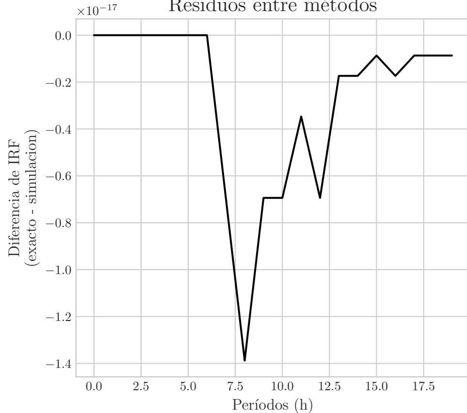
Comparación IRF de un Proceso AR(20)
