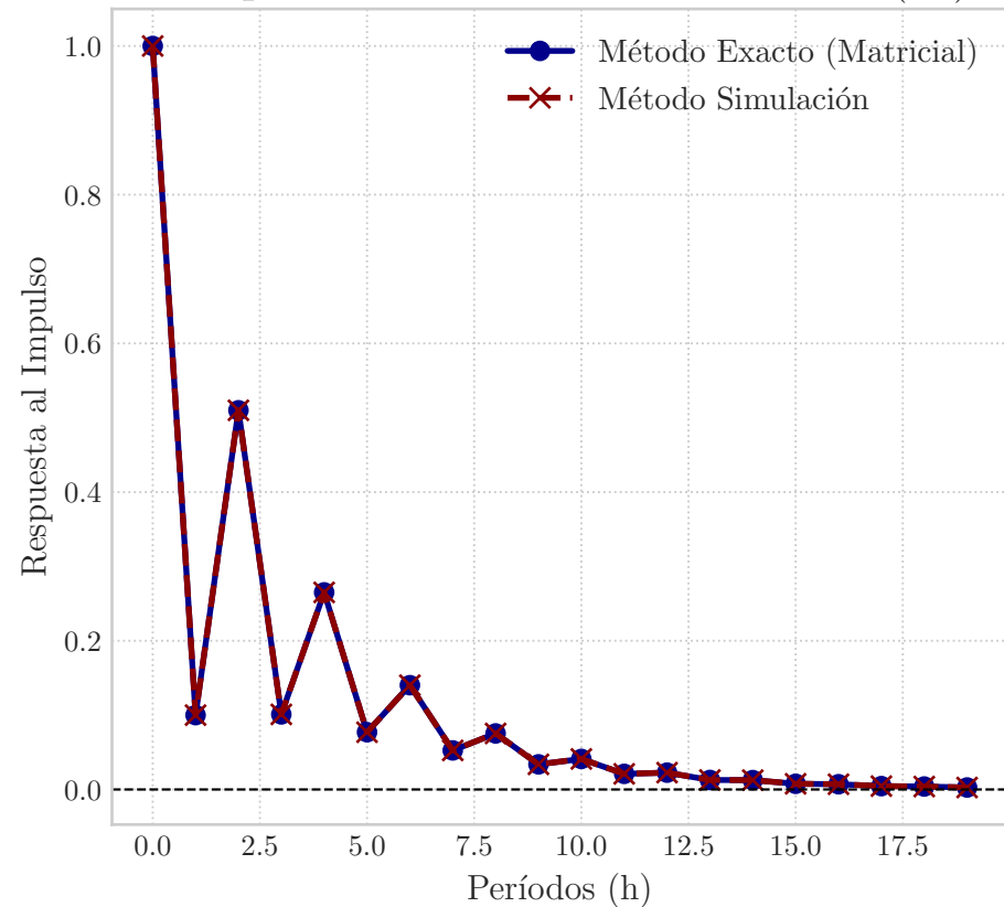
Comparación IRF de un Proceso AR(20)
