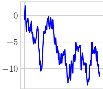
unit_root
