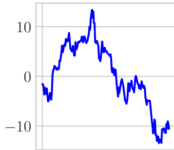
nonlinear_trend
