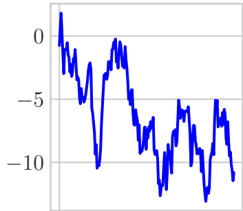
unit_root
