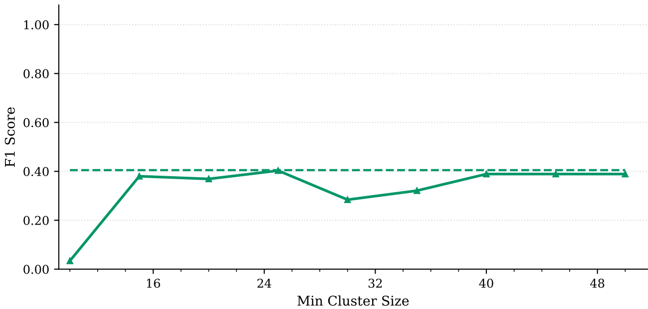
F1 Score
