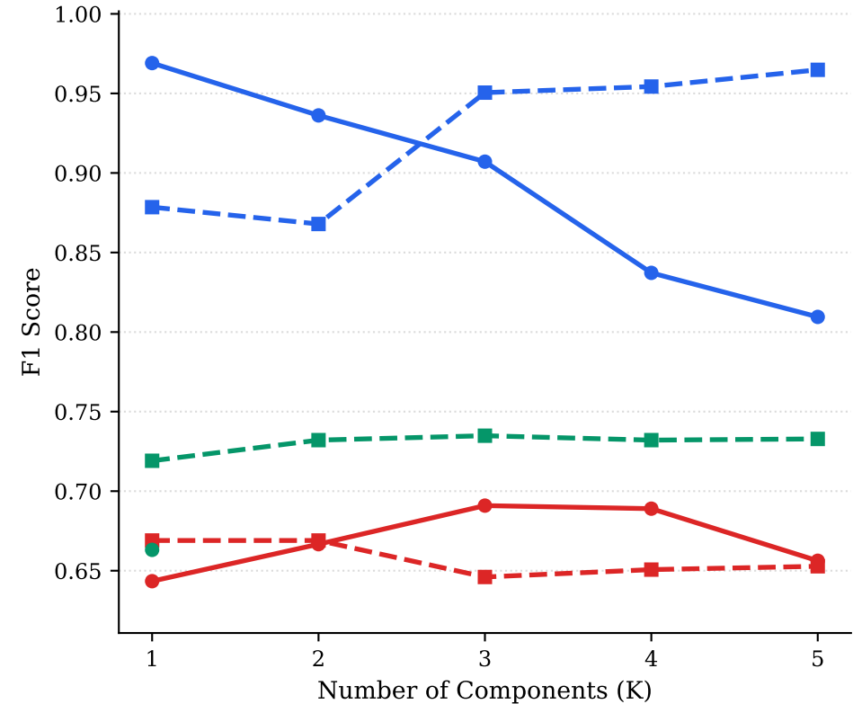
F1 Score
