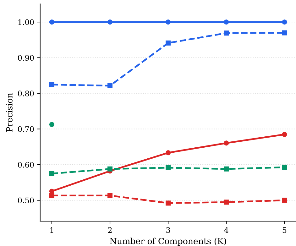
Precision
