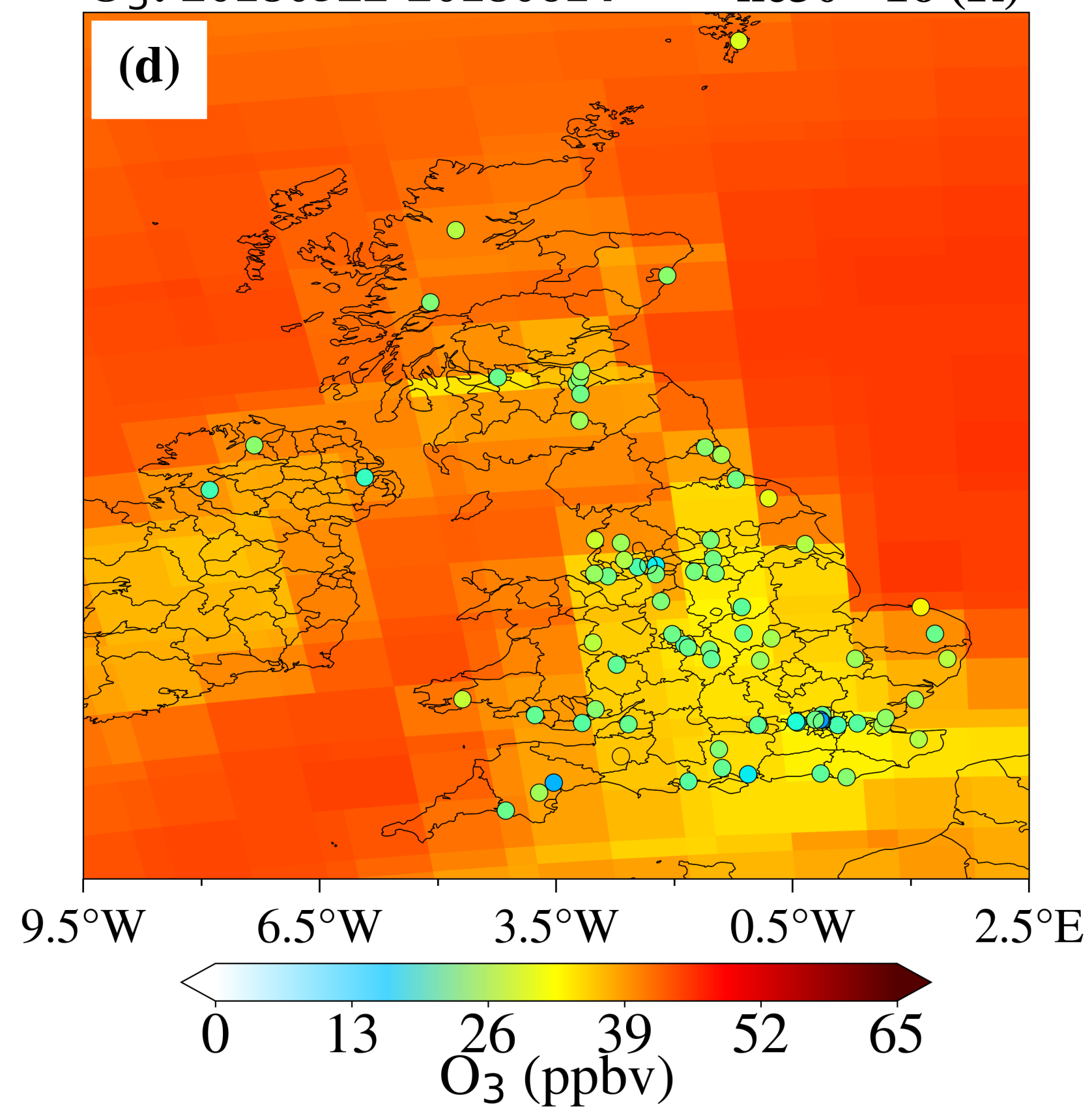
O 3 : 20180522-20180614 ne30×16 (R)
