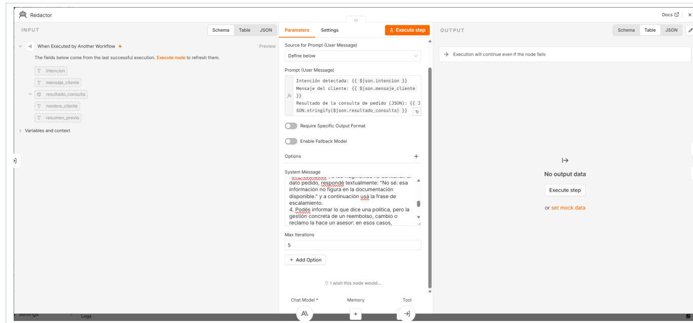
Figura 3. System Message del agente Redactor (Worker 2), con la regla 3 (RAG, citación y «No sé») y la regla 4 (escalamiento de gestiones).
