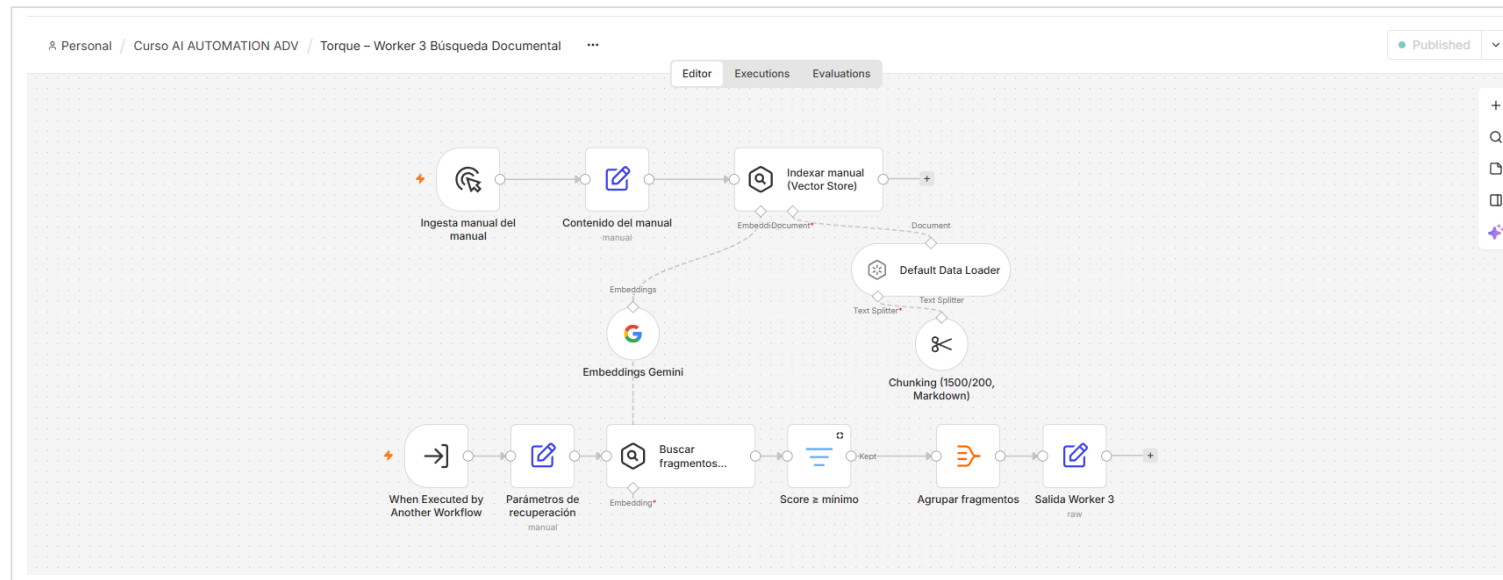
Figura A2.1. Worker 3 - Búsqueda Documental: rama de ingesta (arriba) y rama de recuperación (abajo), con embeddings compartidos.
