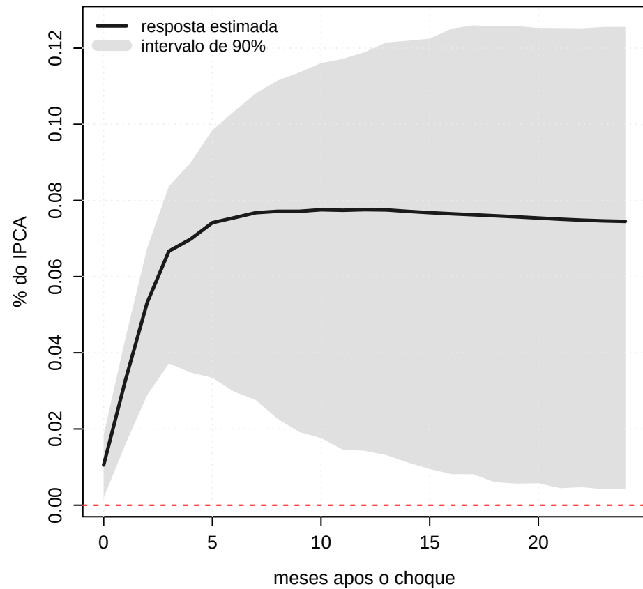
Choque de 1% nas commodities (resposta acumulada)
