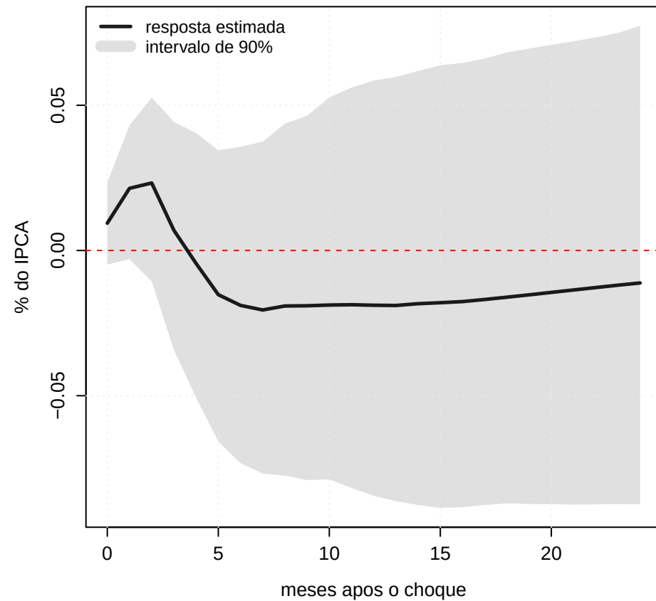
Choque de 1% nos precos de importacao (resposta acumulada)
