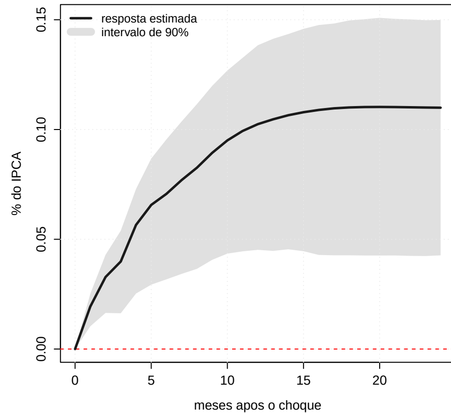
Depreciacao cambial de 1% (resposta acumulada)
