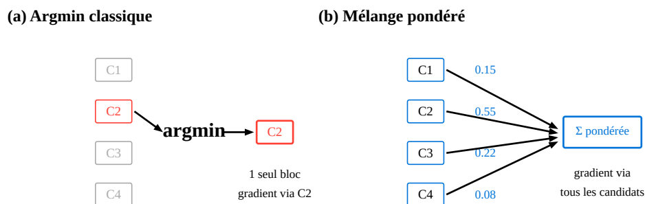
Fig. 24. – Deux façons de gérer la sélection de bloc non différentiable. À gauche, le STE garde le choix dur ( argmin ) et ne propage le gradient que par le bloc gagnant. À droite, notre approche par mélange pondéré ( softmax ) combine tous les candidats selon leur pertinence, laissant le gradient circuler à travers chacun.
