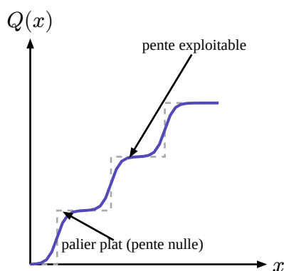
Fig. 26. – Arrondi dur (escalier, en pointillés) et sa version adoucie continue ( soft round ).
