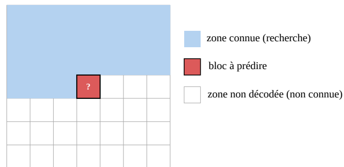
Fig. 25. – Zone de recherche causale pour la prédiction d'un bloc. Seule l'information déjà décodée (au-dessus et à gauche) est disponible.
