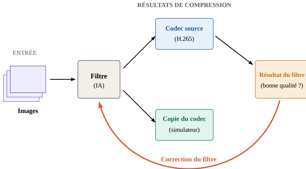
Fig. 23. – Déroulement de la boucle d'apprentissage du filtre
