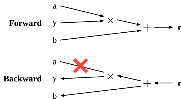
Fig. 22. – Graphe de calcul : r = ay + b ( a est détaché, son gradient est bloqué au backward )
