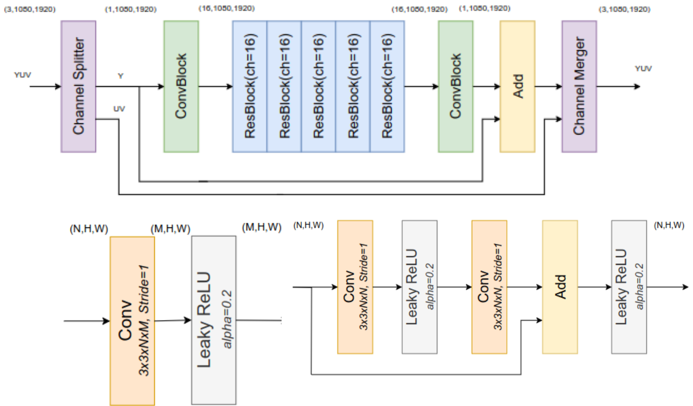
Fig. 39. – Architecture du réseau et ses briques de base : architecture globale (haut), en bas, convblock (gauche) et resblock (droite). [13]
