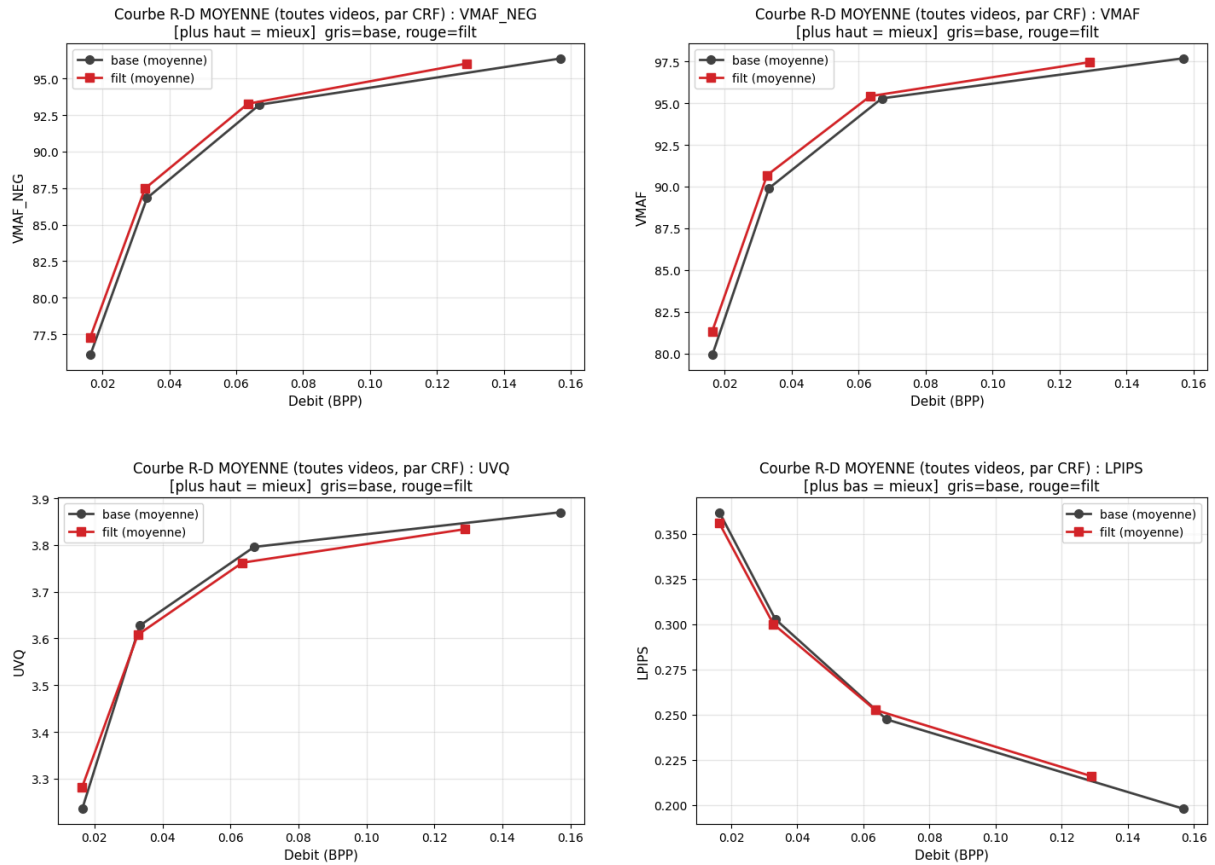
Fig. 28. – Résultats Optimisation filtre avec proxy simplifié version « arrondi »
