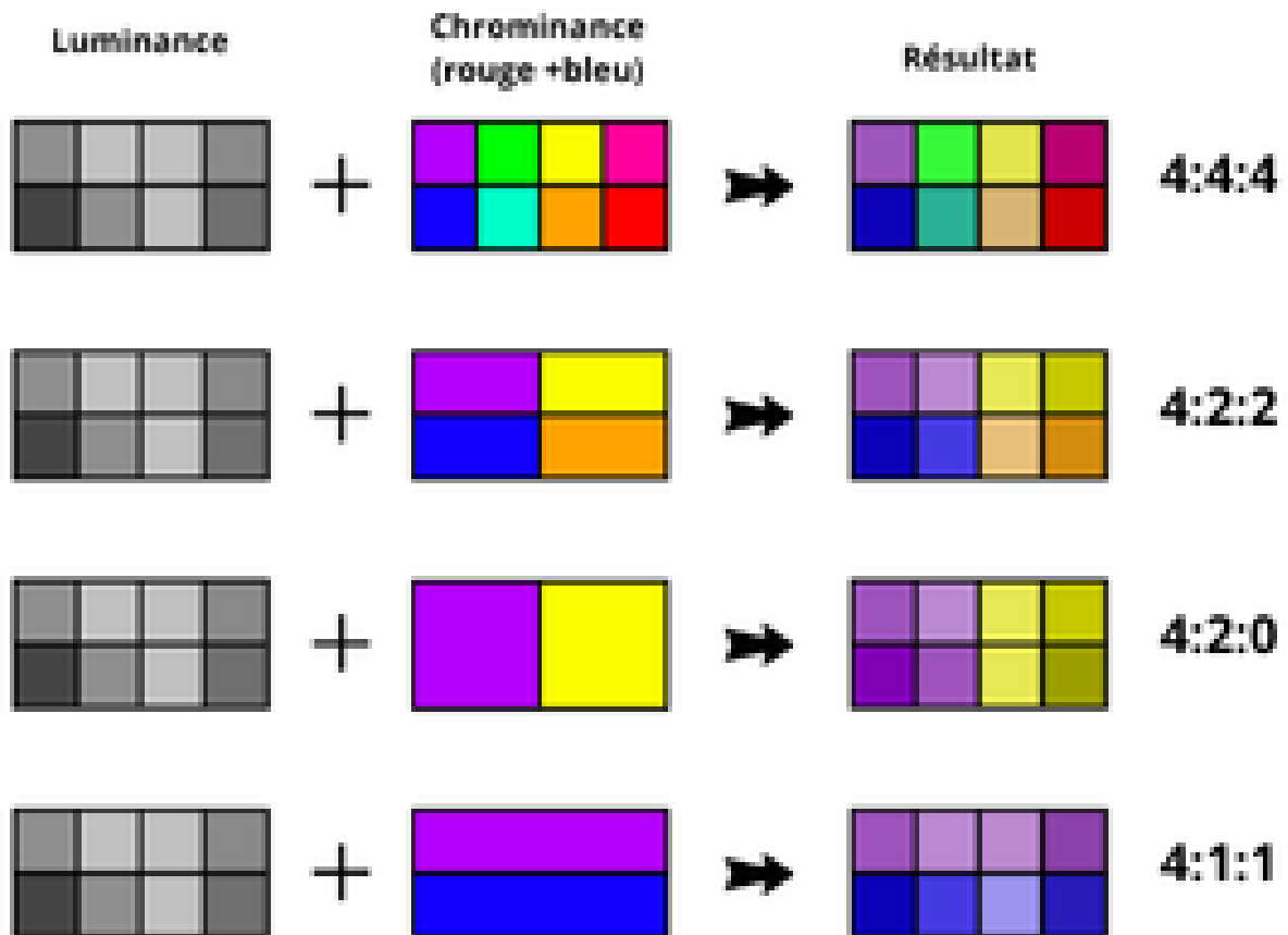
Fig. 17. – Exemple de réduction des données en 4:2:0 et autres formats, [12]
