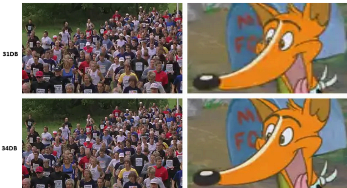
Fig. 19. – Exemple de la différence entre fidélité structurelle et qualité perçue (score PSNR de 31 dB, mauvais, pour les deux images du haut, et de 34 dB, meilleur, pour celles du bas)
