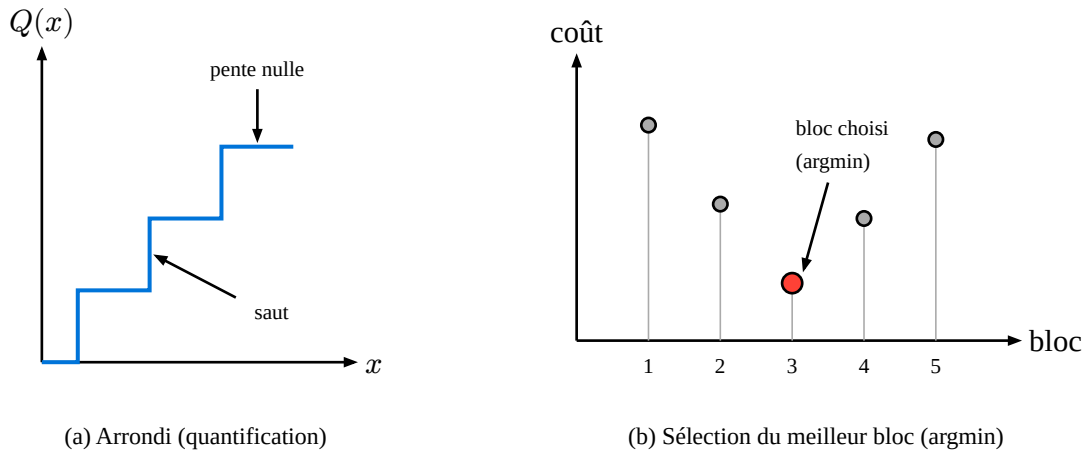
Fig. 21. – Deux opérations non différentiables typiques d'un codec . À gauche, l'arrondi de la quantification : sa courbe en escalier est plate entre les marches et discontinue aux sauts. À droite, la sélection du meilleur bloc par argmin : le choix n'est pas continu, il saute d'un bloc à l'autre sans fournir de pente exploitable.
