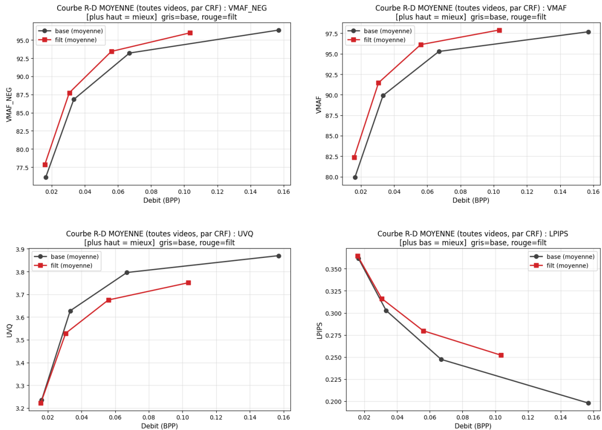
Fig. 27. – Résultats Optimisation filtre avec proxy neuronal
