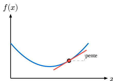
Fig. 20. – Cas d'une fonction différentiable : en tout point, on peut calculer la pente (le gradient), qui indique dans quel sens la fonction varie, et donc dans quelle direction ajuster le paramètre.
