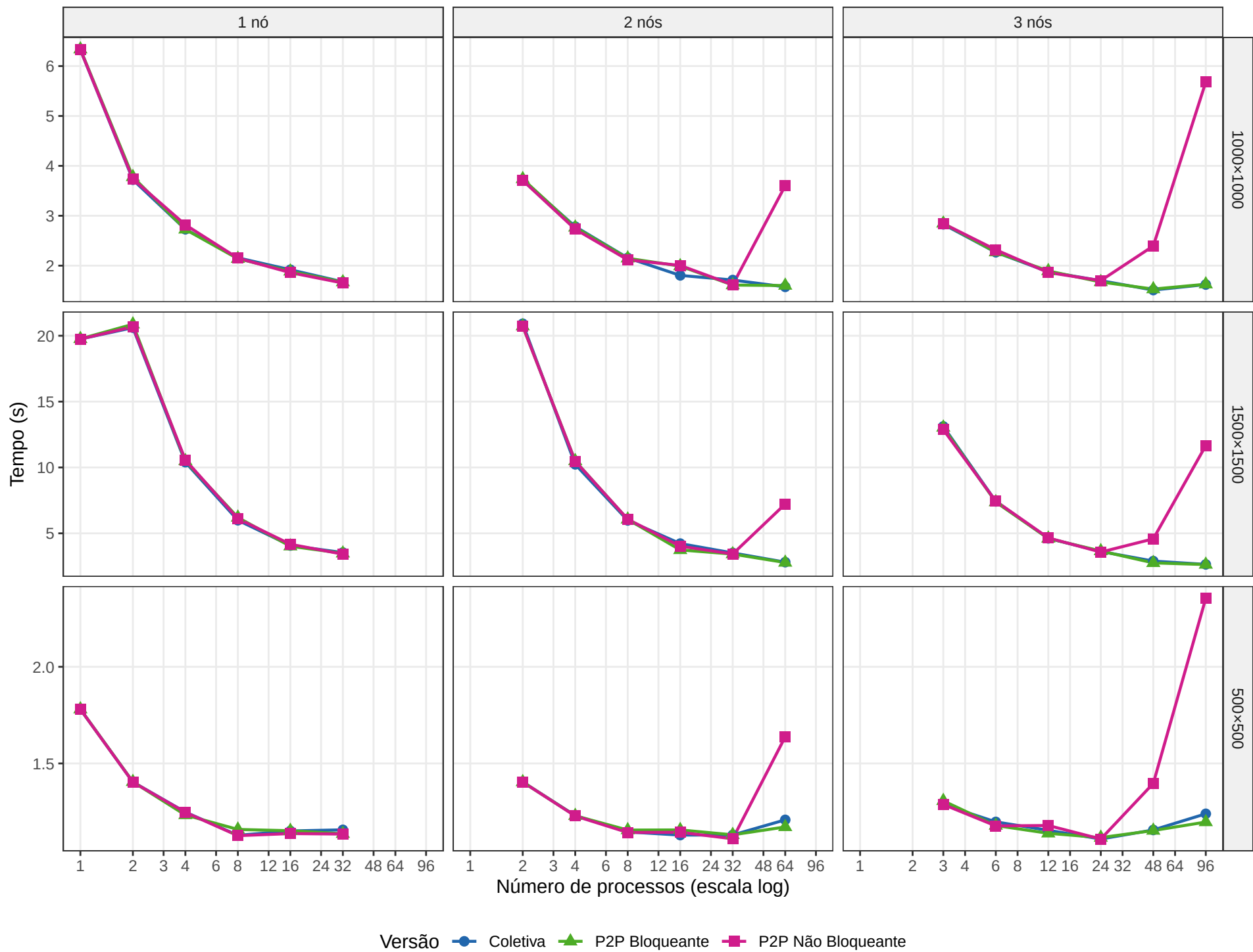
Tempo total de execução (mediana de 2 repetições)
