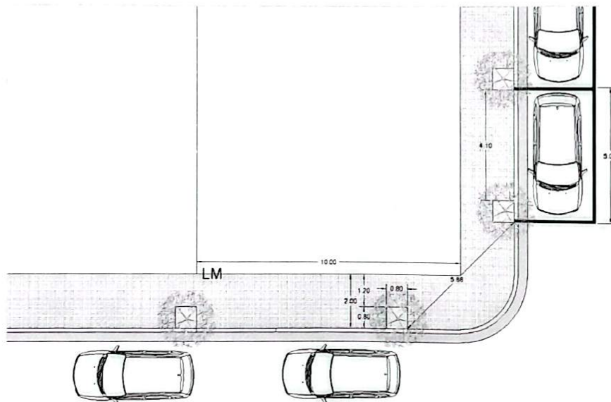
Figura 1 – Ubicación de canteros en veredas de mas de 2 m.
