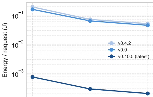
Online Boutique
