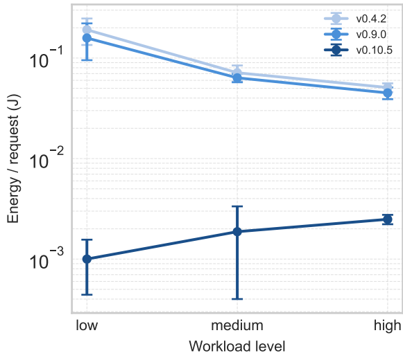
onlineboutique
