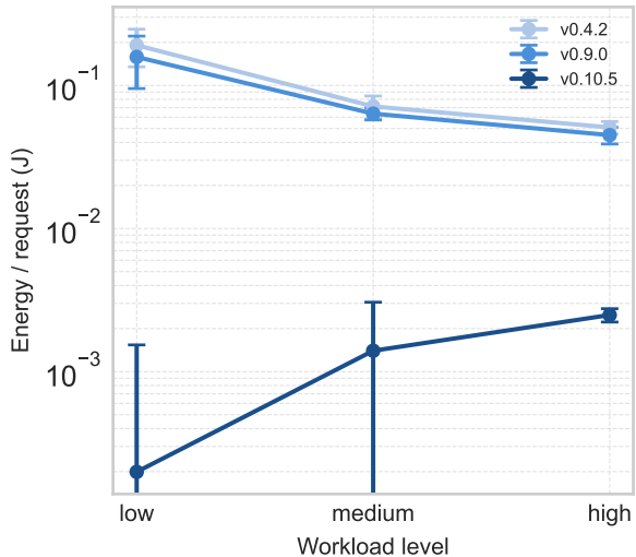
onlineboutique
