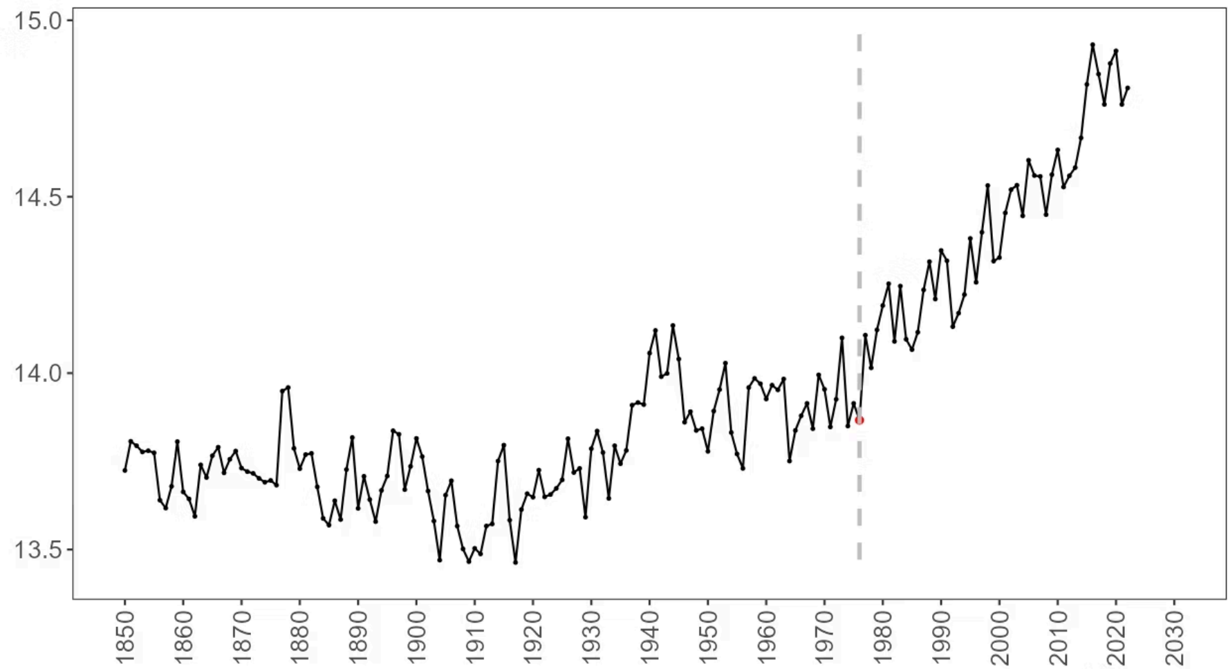
Linhas tracejadas indicam pontos de mudança detectados com estatística de Chow.
