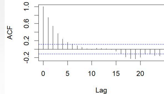
ACF: dependência temporal AR(1)
