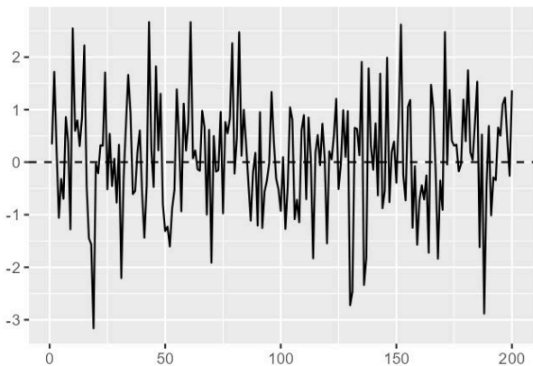
Ruído: flutuações aleatórias
