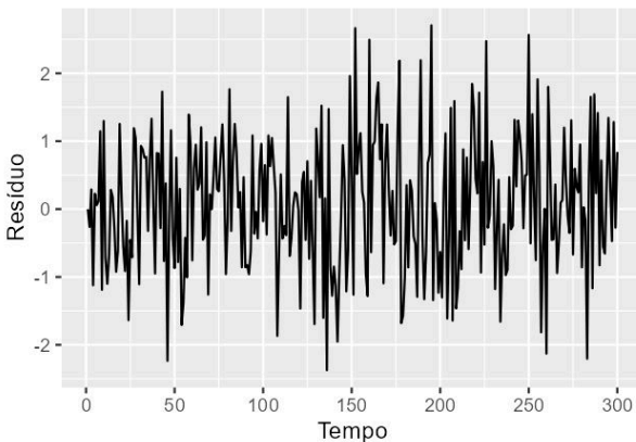
Resíduos do ARIMA (ideal: ~ ruído branco)
