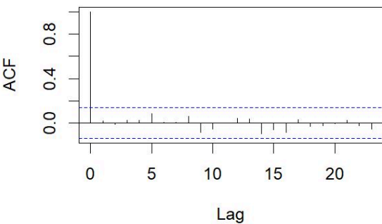
ACF do ruído branco (esperado ~ 0)
