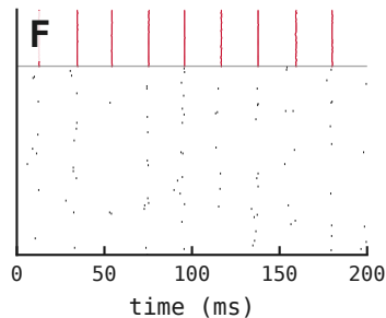
W EI =3.0, W IE =6.0 contrast=0.98
