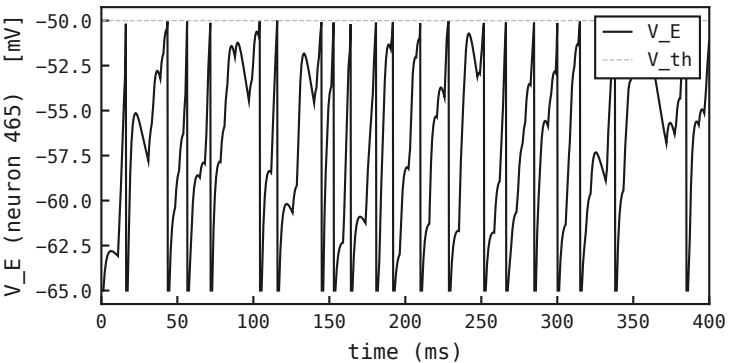
COBA · E-neuron membrane voltage
