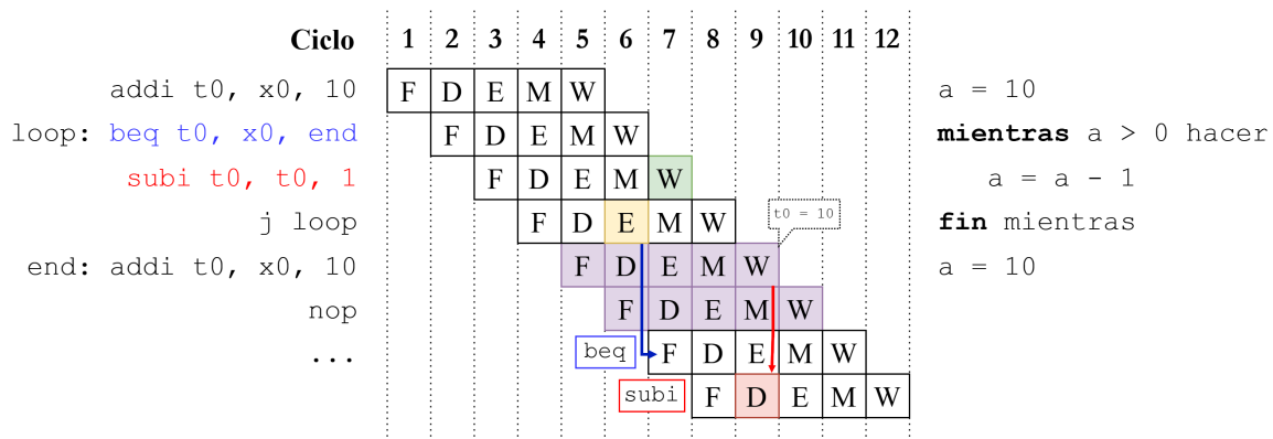
Figura 5.3: Representación del flujo de ejecución de un programa sobre una arquitectura segmentada sin mecanismos para resolver riesgos de control. Nótese que el resultado de la instrucción de resta ( subi ) se escribe (writeback señalado en color verde) en el banco de registros ántes incluso de evaluar la condición en la instrucción de salto, dejando el valor del registro t0 en un estado inconsistente. Además, dado que el destino del salto de la instrucción jal no se calculará hasta su ejecución, habrá dos ciclos en los que se introducirán las dos instrucciones inmediatamente posteriores (señaladas en color morado), una de las cuales reinicia el valor de la variable a haciendo que el bucle no tenga final. El resultado de la instrucción subi en la primera iteración se sobrescribe con el del segundo addi .
