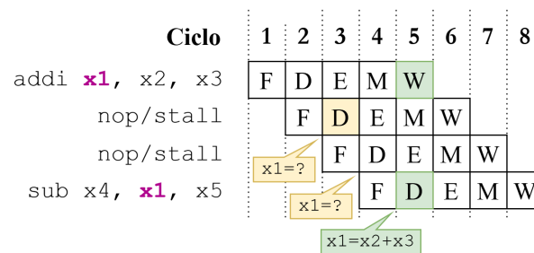
Figura 5.3: Flujo de ejecución de dos instrucciones implicadas en una dependencia RAW. Se señala en color verde el instante a partir del cual la segunda instrucción podrá leer el dato actualizado en el registro x1 (ciclo 5).
