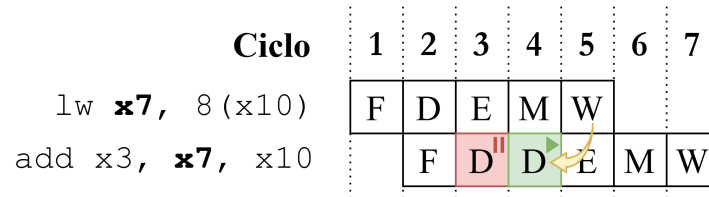
Figura 5.15: Flujo de ejecución de dos instrucciones implicadas en una dependencia de datos de tipo RAW, una de las cuales es la instrucción lw .
