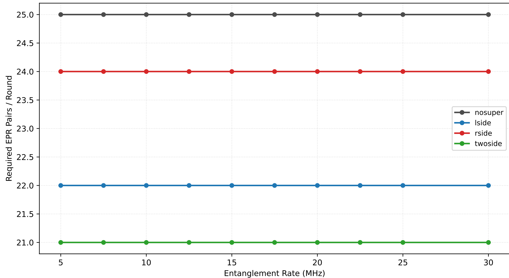
Raw Pairs Sweep d=13 k=6 rounds=14 shots=500000
