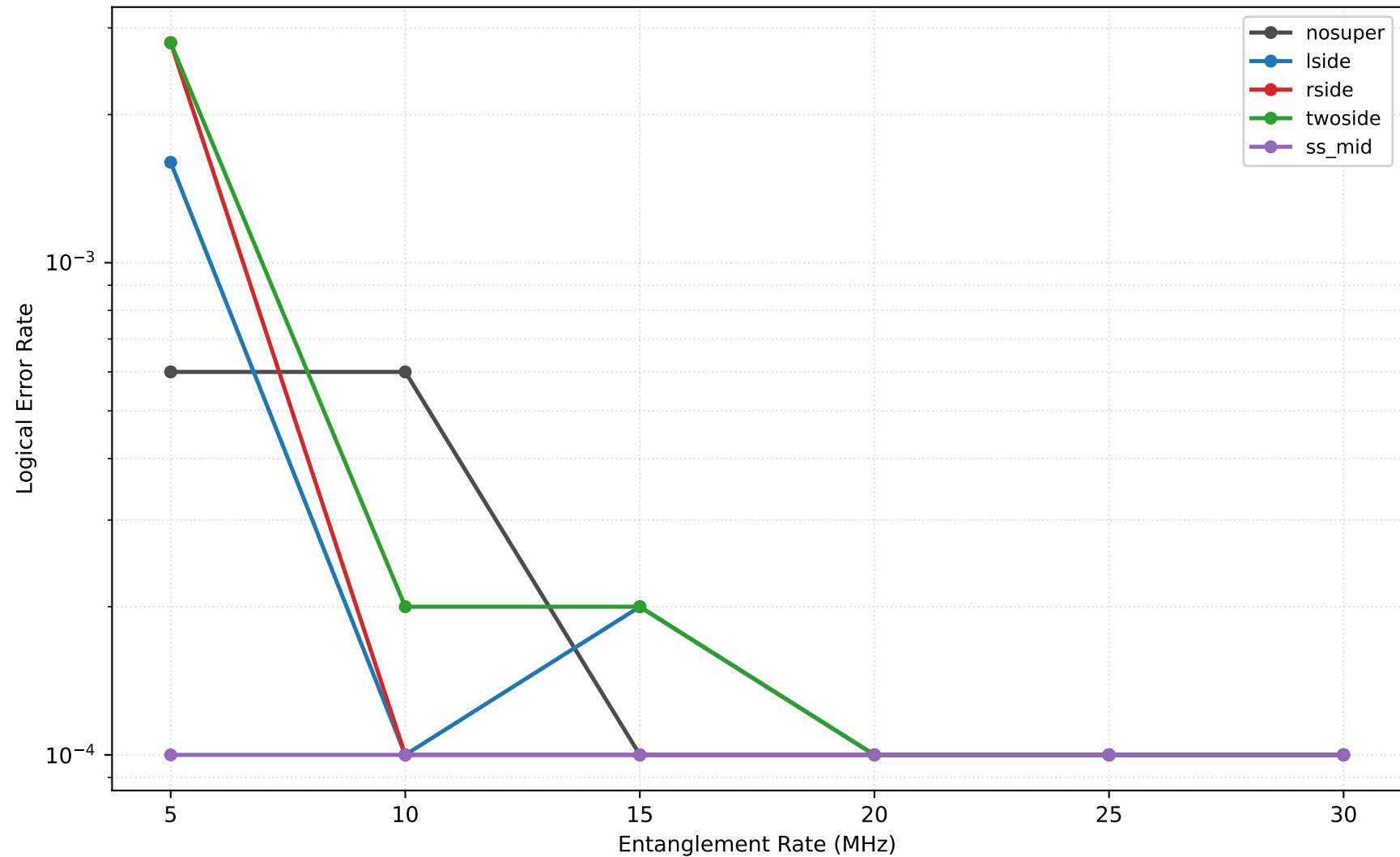
Raw Pairs Sweep d=13 k=6 rounds=6 shots=5000
