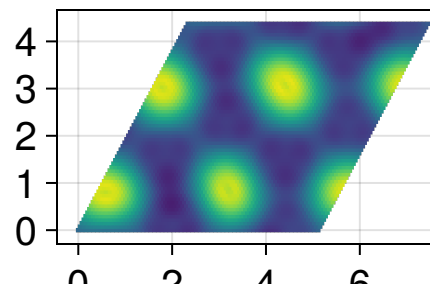
l. PBE
