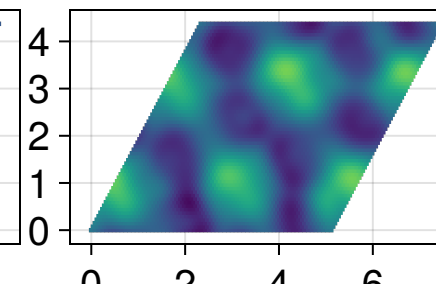
m. FNO
