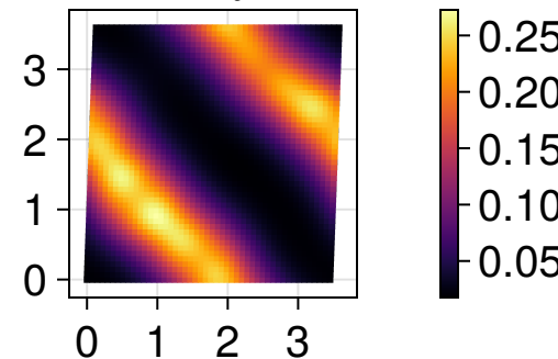
f. Density
