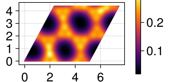
o. Density
