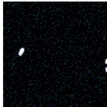
DDRM Reconstruction
