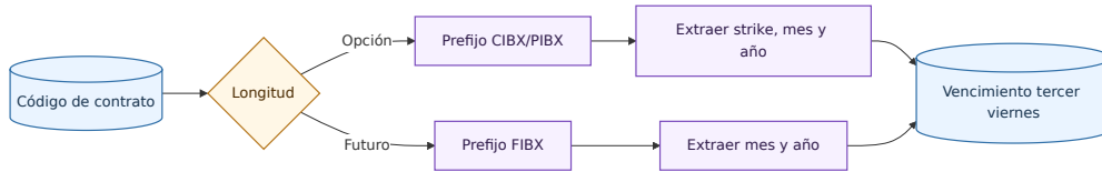
Figura 16: Validacion e interpretacion del codigo de contrato.
