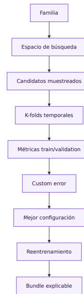
Figura 20: Selección de modelos mediante k-folds temporales.
