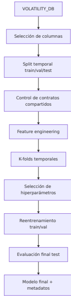
Figura 22: Flujo de modelización de volatilidad.
