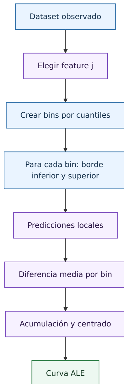
Figura 43: Construcción de curvas ALE por bins locales.
