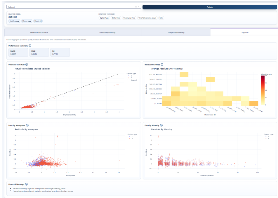
Figura 28: Diagnosis en XGBoost.
