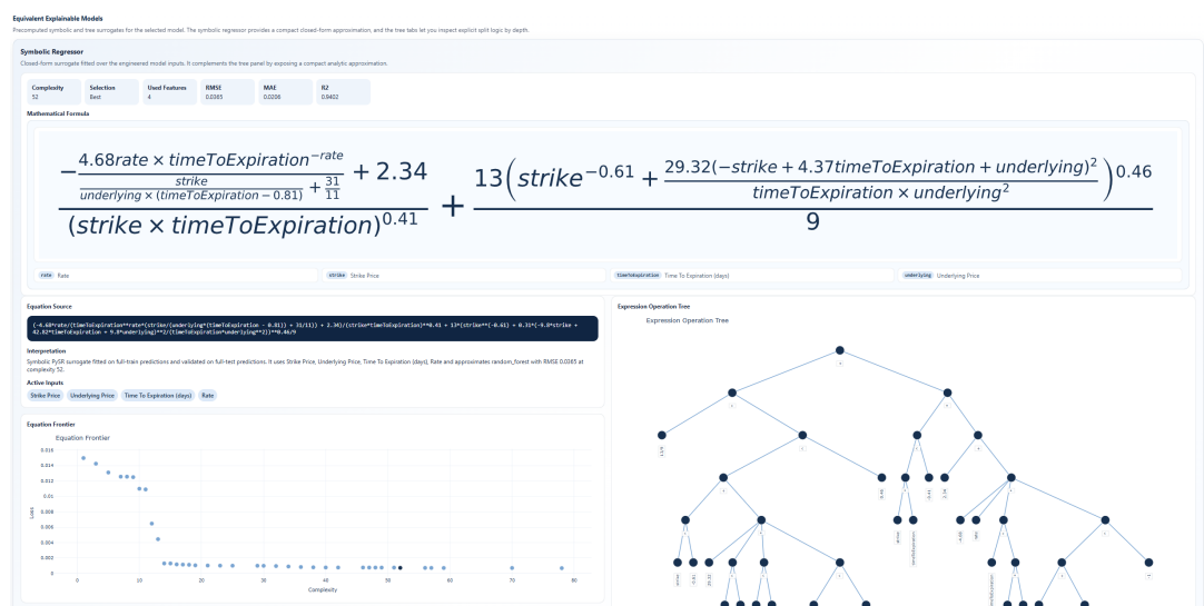
(b) Regresión simbólica de Random Forest.
