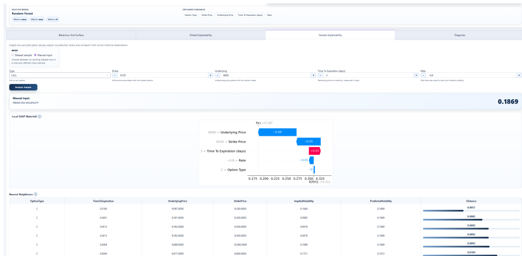
Figura 33: Explicabilidad local en modo manual input (stress corto vencimiento) en Random Forest: contraste de coherencia local y soporte histórico.
