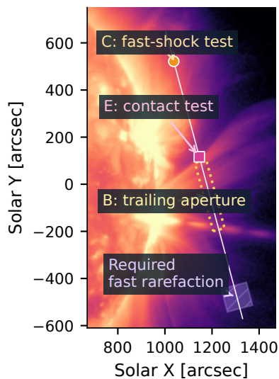
(a) SUVI 195 Å | 15:58:24.76 UT
