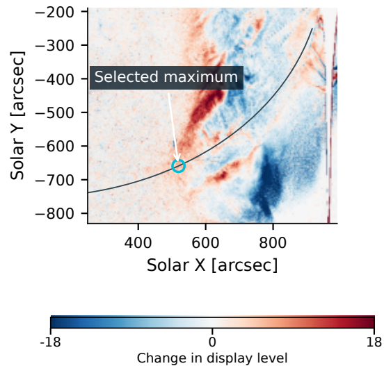
(d) AIA 193 Å | 10 September 2017
