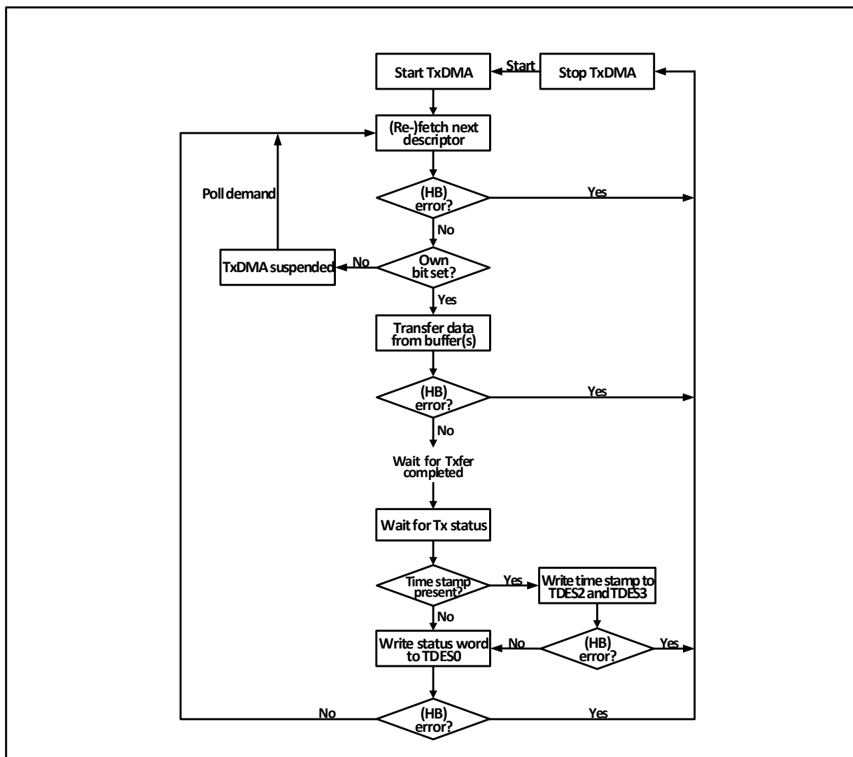
图 27-11 发送流程
