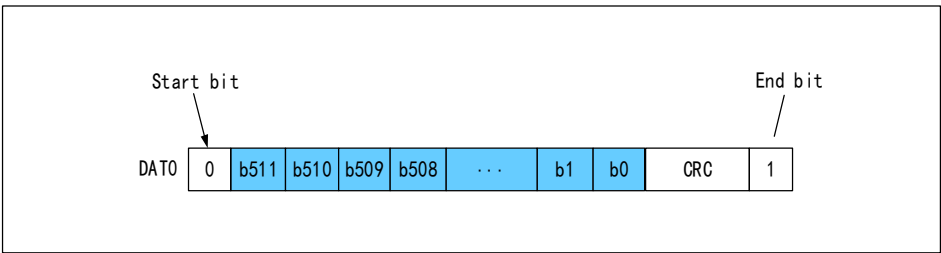
图 28-11 SD 卡单总线数据传输一个 512 位字的格式
