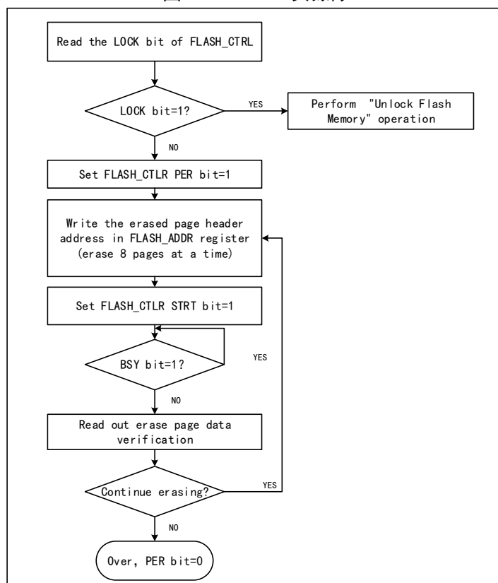
图 32-2 FLASH 页擦除
