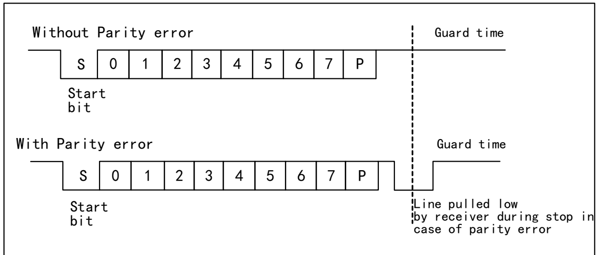
图 18-4 （未）发生奇偶校验错误示意图
