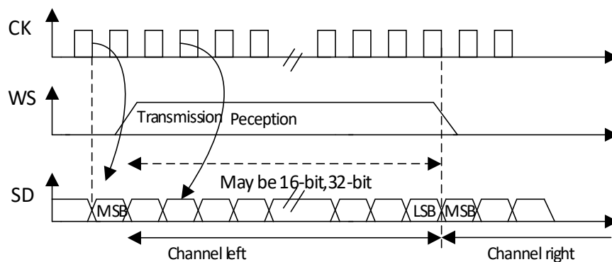
图 20-10 LSB 对齐 16 或 32 位全精度, CPOL = 0
