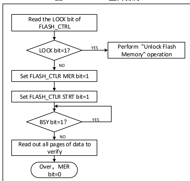
图 32-3 FLASH 整片擦除
