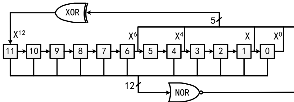
图 17-5 LFSR 寄存器算法
