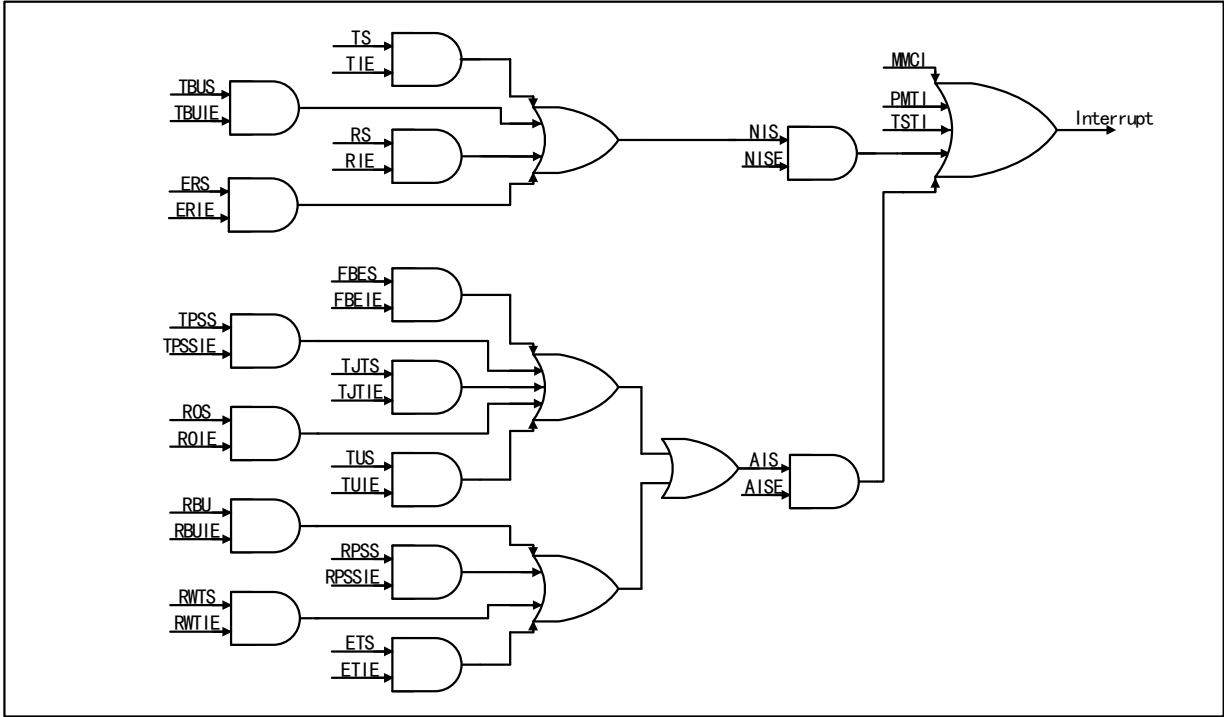
图 27-13 中断示意图
