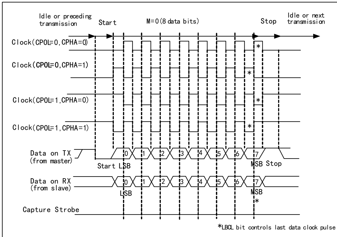
图 18-3 数据采样保持时间
