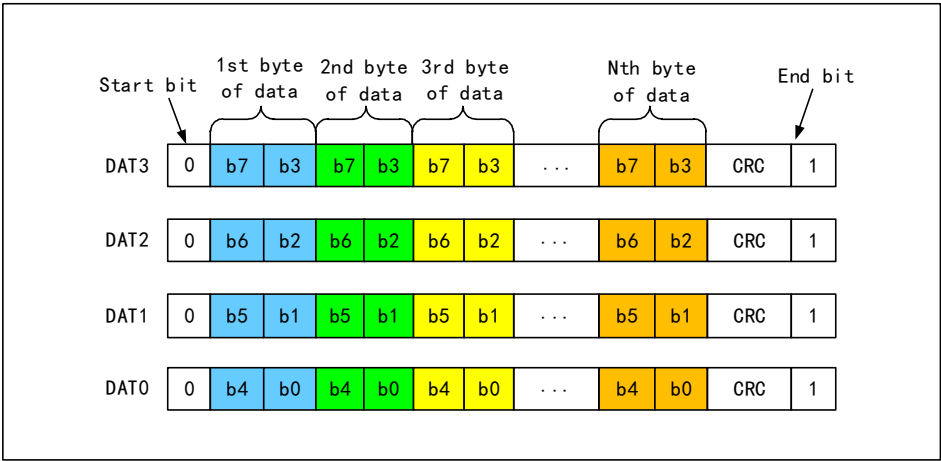
图 28-10 SD 卡 4 总线数据传输字节的格式
