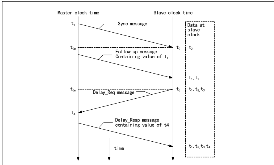
图 27-9 IEEE1588 PTP 协议同步报文时序图
