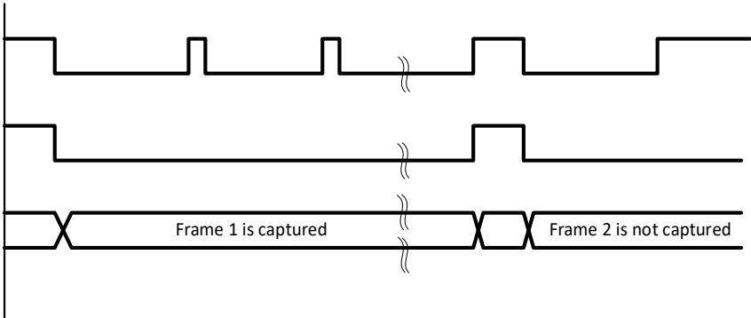
图 25-3 快照模式下的单帧捕获波形
