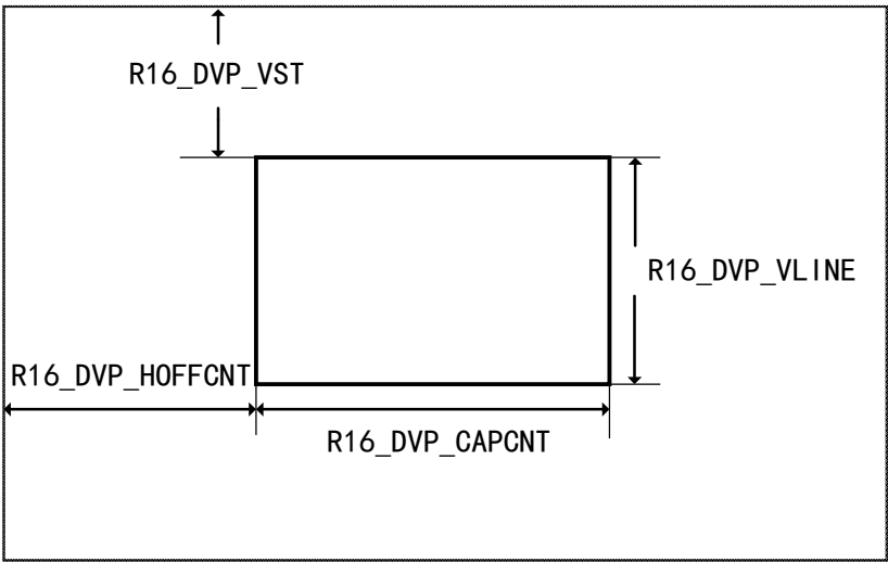
图 25-5 裁剪窗口的坐标和大小
