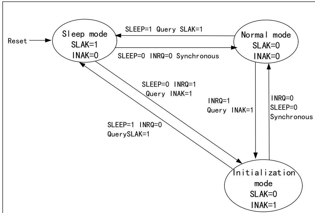
图 24-1 CAN 工作模式切换
