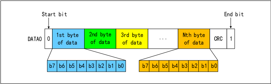
图 28-9 SD 卡单总线数据传输字节的格式
