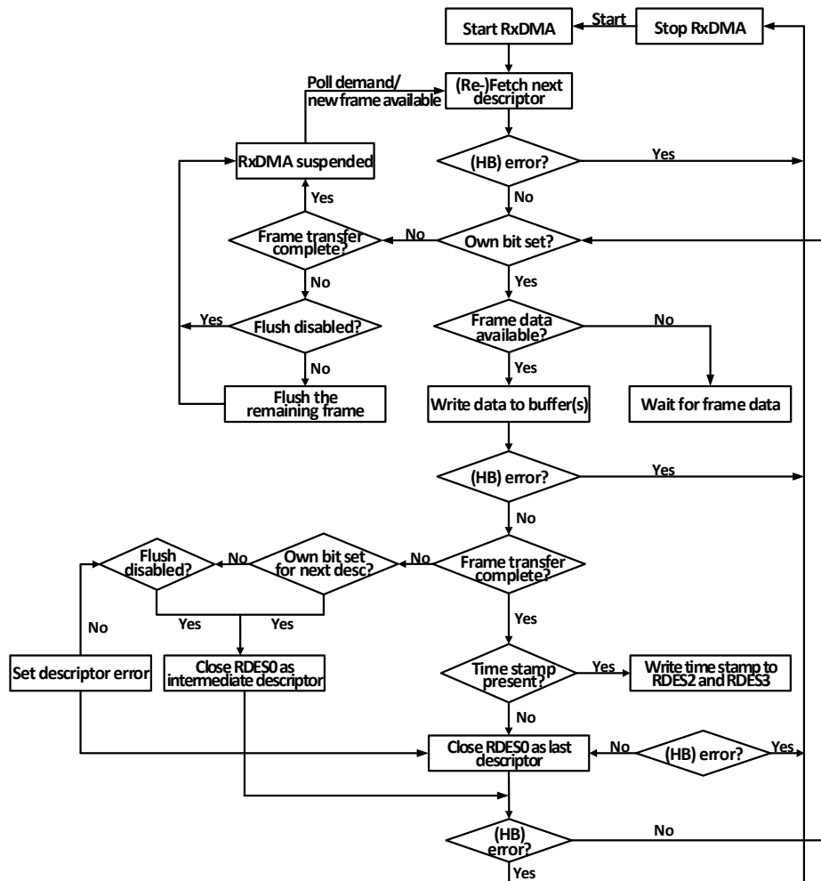
图 27-12 接收流程
