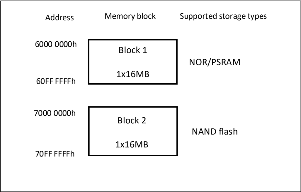
图 26-2 FSMC 存储块
