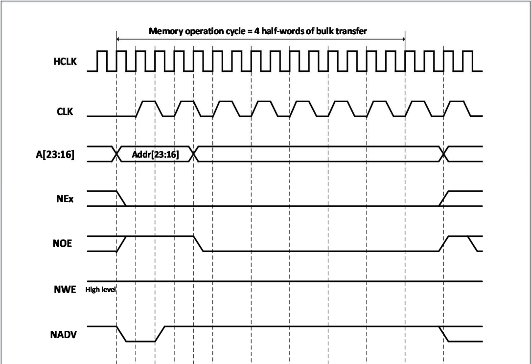
图 26-13 同步总线复用读操作（复用）
