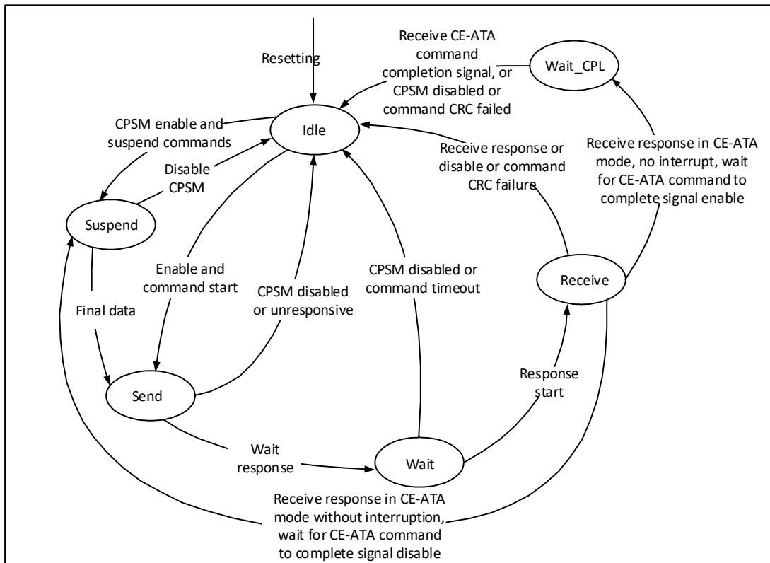
图 28-2 命令状态机
