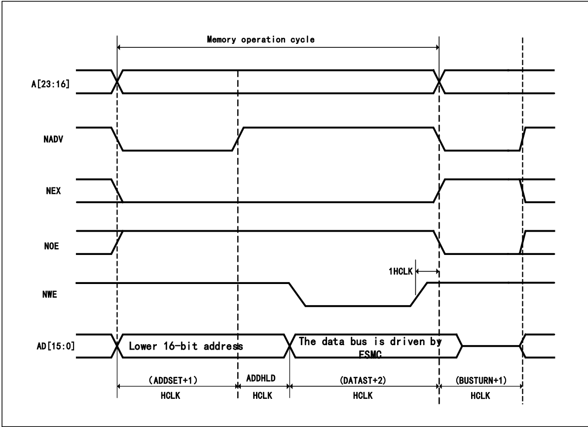
图 26-12 模式 D 写操作（复用）
