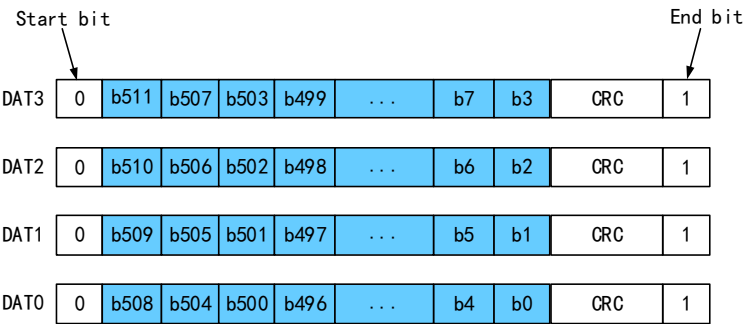
图 28-12 SD 卡 4 总线数据传输一个 512 位字的格式
