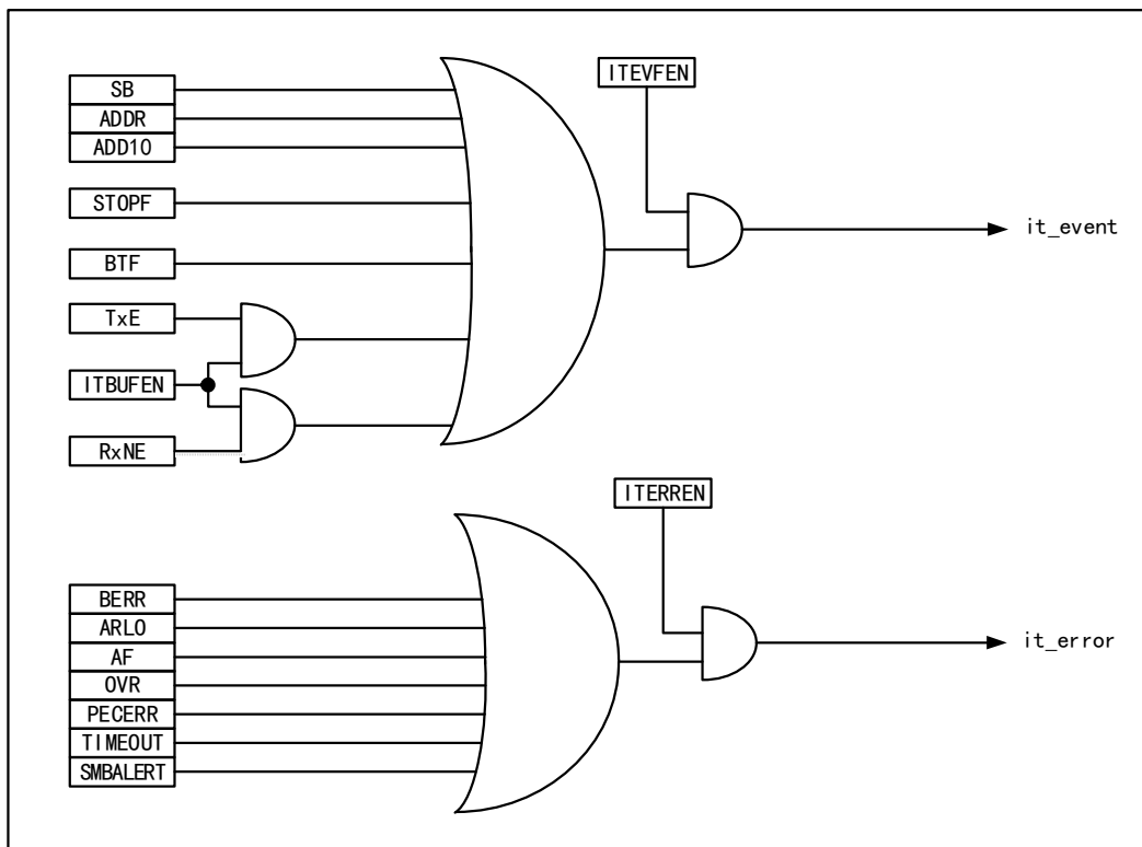
图 19-8 I2C 中断请求
