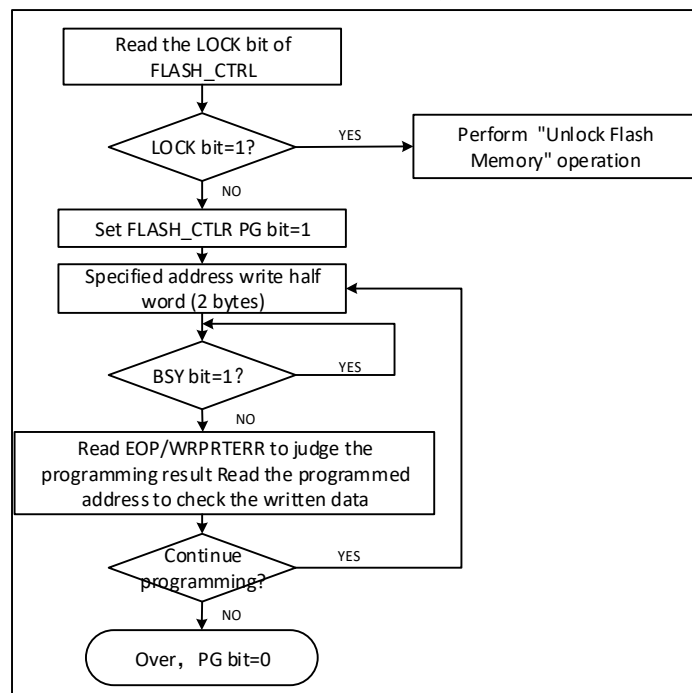
图 32-1 FLASH 编程
