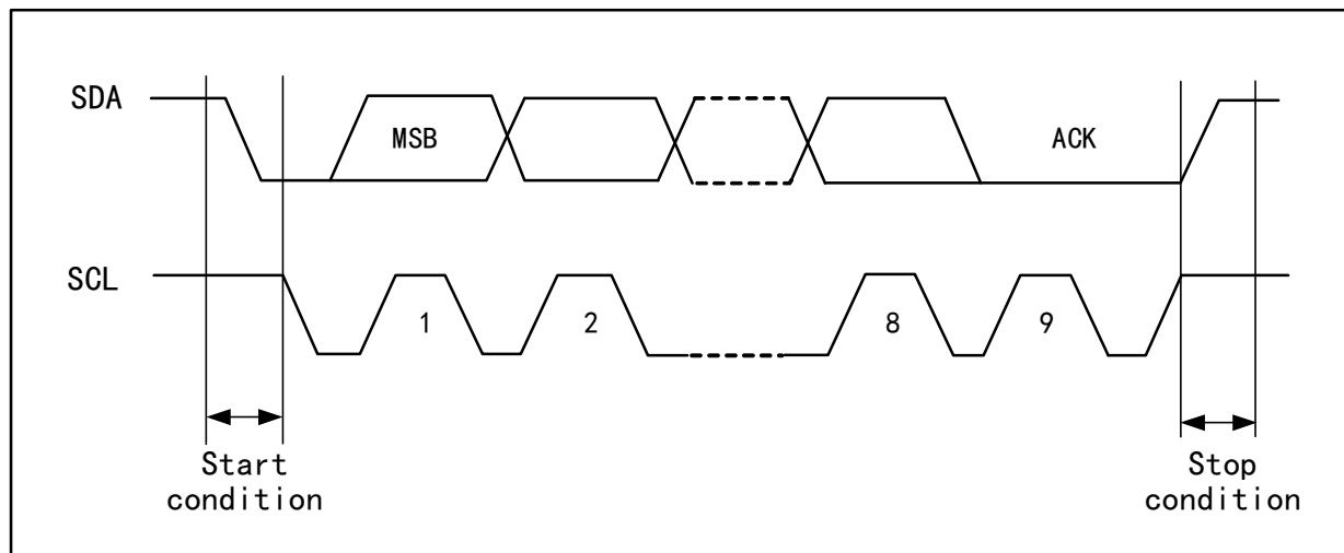
图 19-1 I2C 时序图
