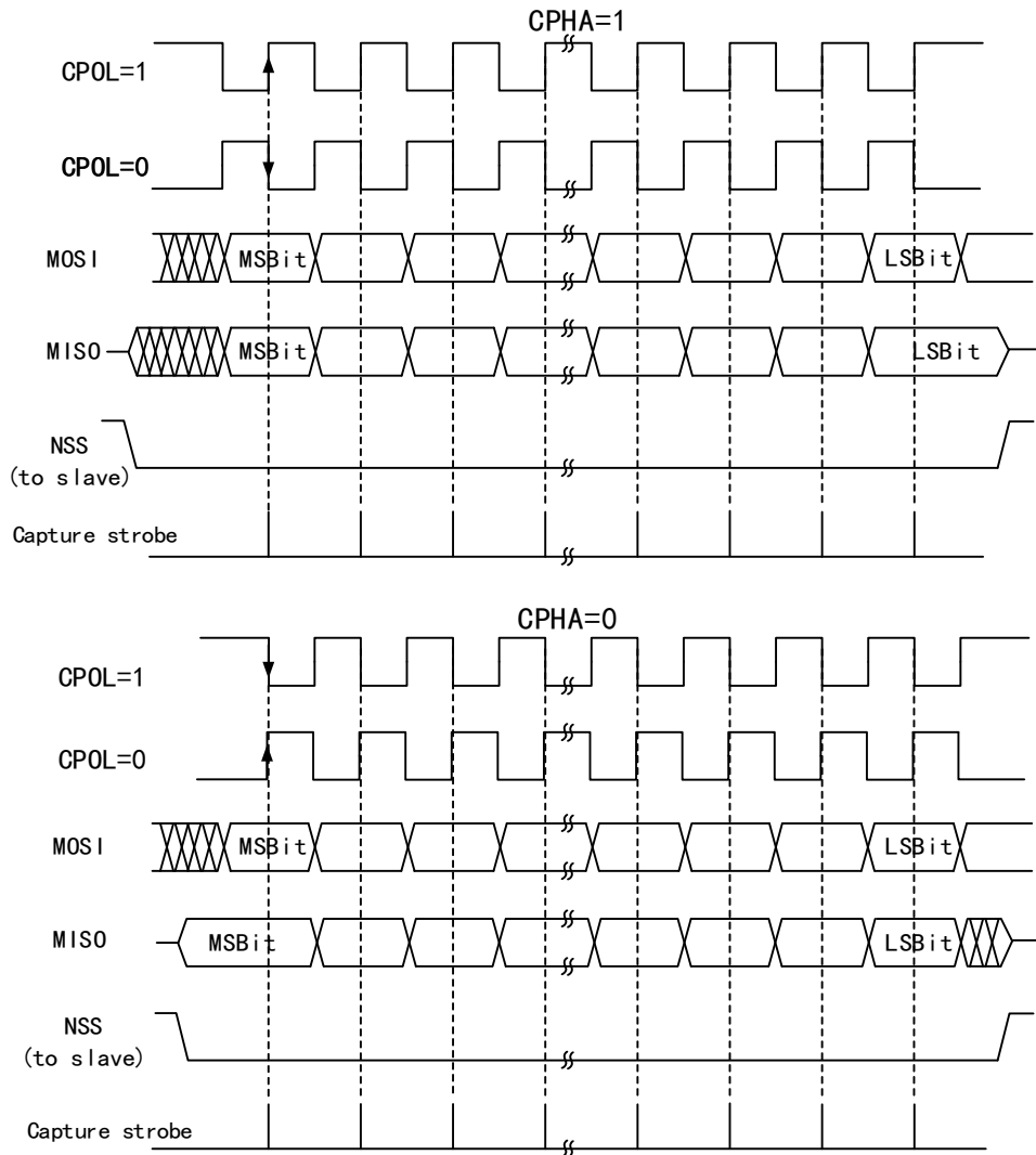
图 20-2 SPI 模式
