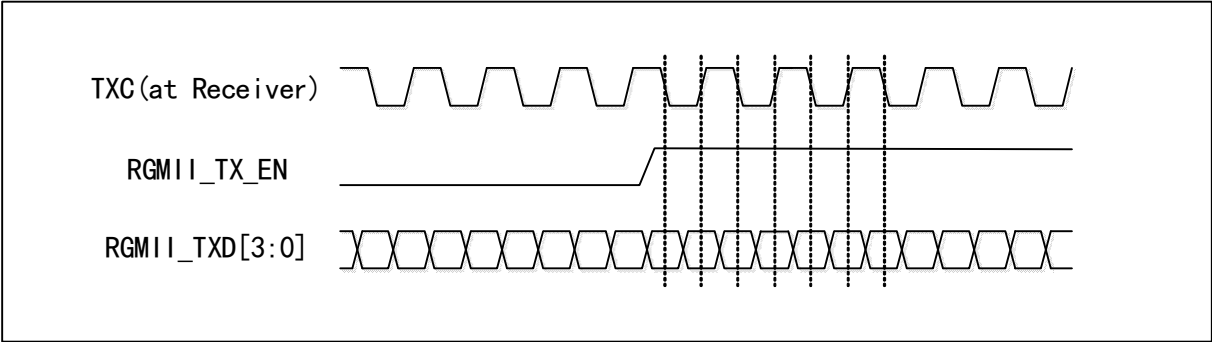
图 27-7 RGMII 的时序示意图
