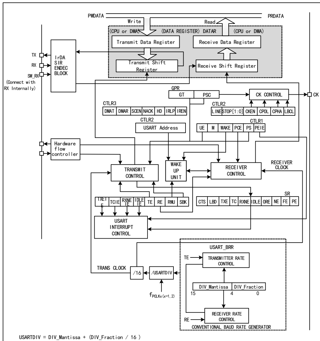
图 18-1 通用同步/异步收发器的结构框图
