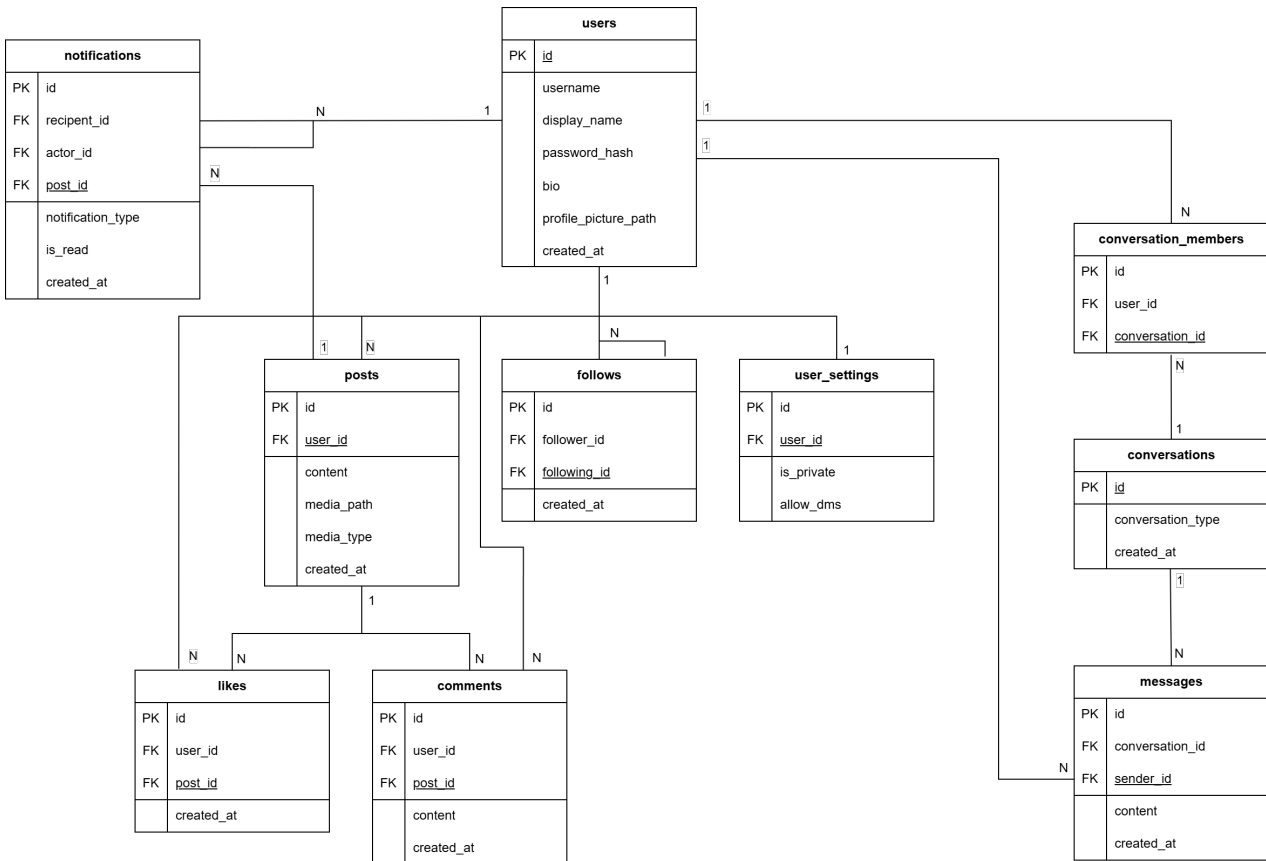
图 4: myownX 系统 ER 图
