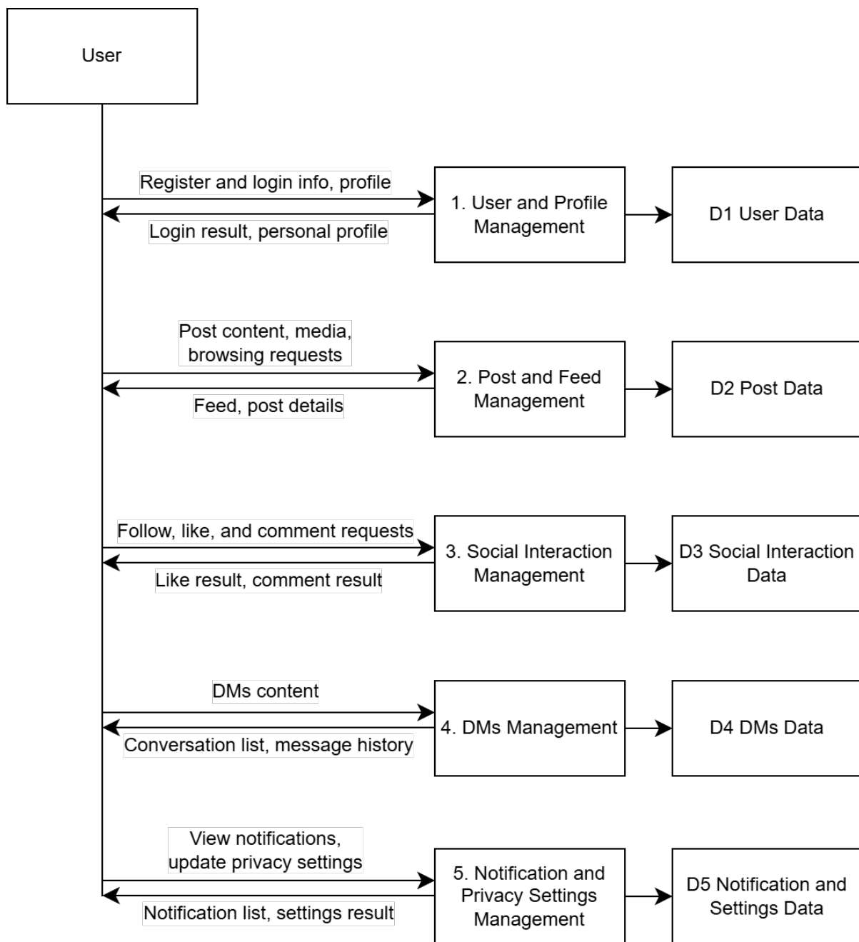
图 3: myownX 社交网络平台 0 层数据流图
