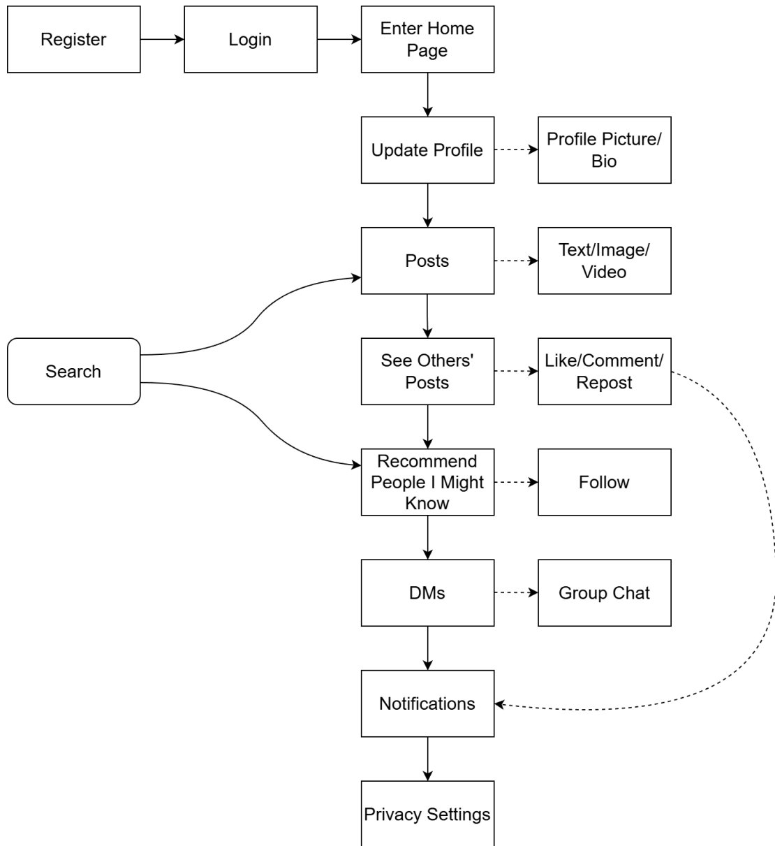
图 1: myownX 用户核心业务流程图
