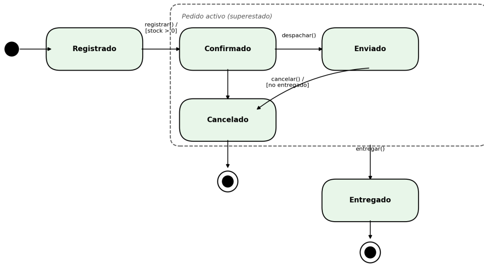
Figura 1: Máquina de estados UML del ciclo de vida de un Pedido.
