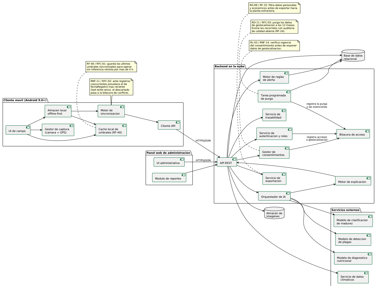
Figura 12: Diagrama de componentes del SIMPA.
