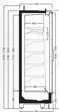
LION V2 PGD/75/220-205
