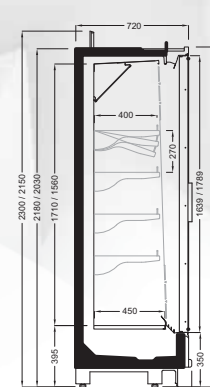
LION V2 PGD/75/220-205
