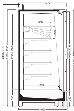
LION V2 PGD/110/220-205
