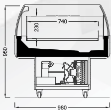
SPIDER 1000/1050
