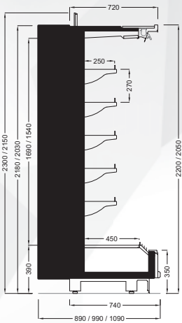
LION CC 75 /90-100-110/ 220-205
