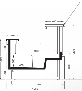
KANGAROO V1 900 FG/CB
