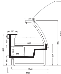
KANGAROO V1 800 FG/CB
